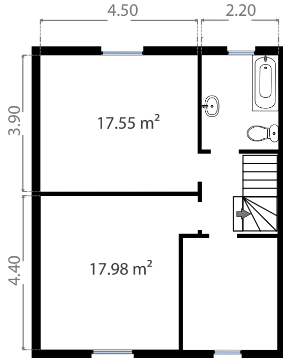
1e Verdieping
