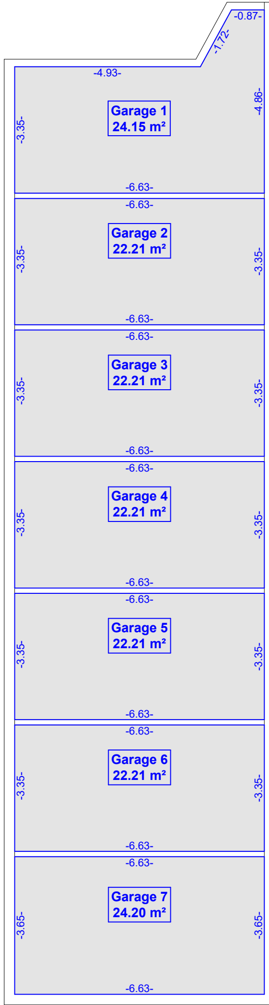
Gelijkvloers - Garages
