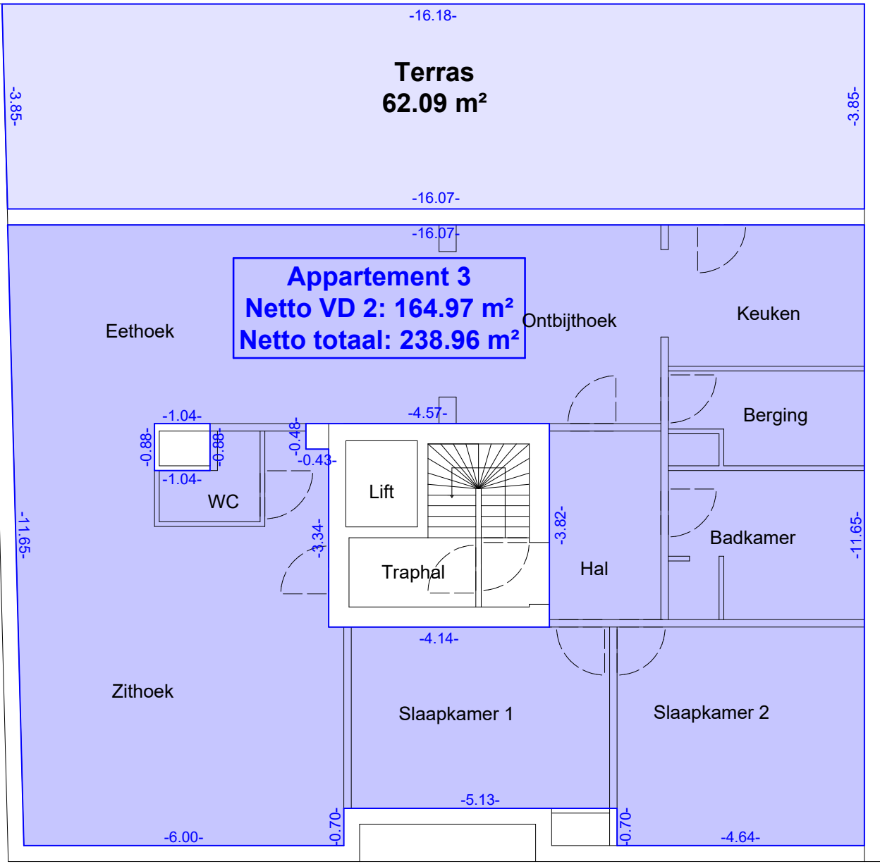
2de Verdieping
