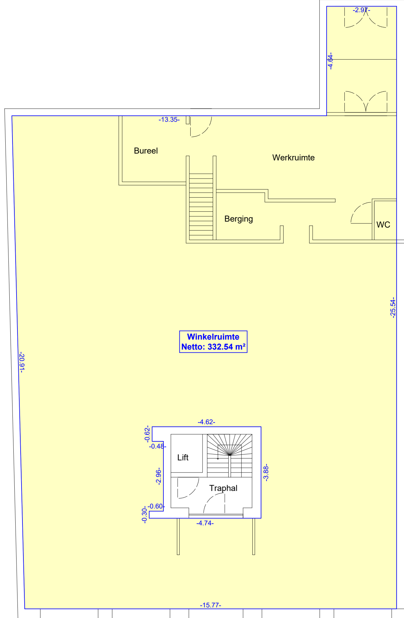
Gelijkvloers - Winkelruimte
