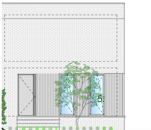
WONING 1: voorgevel
