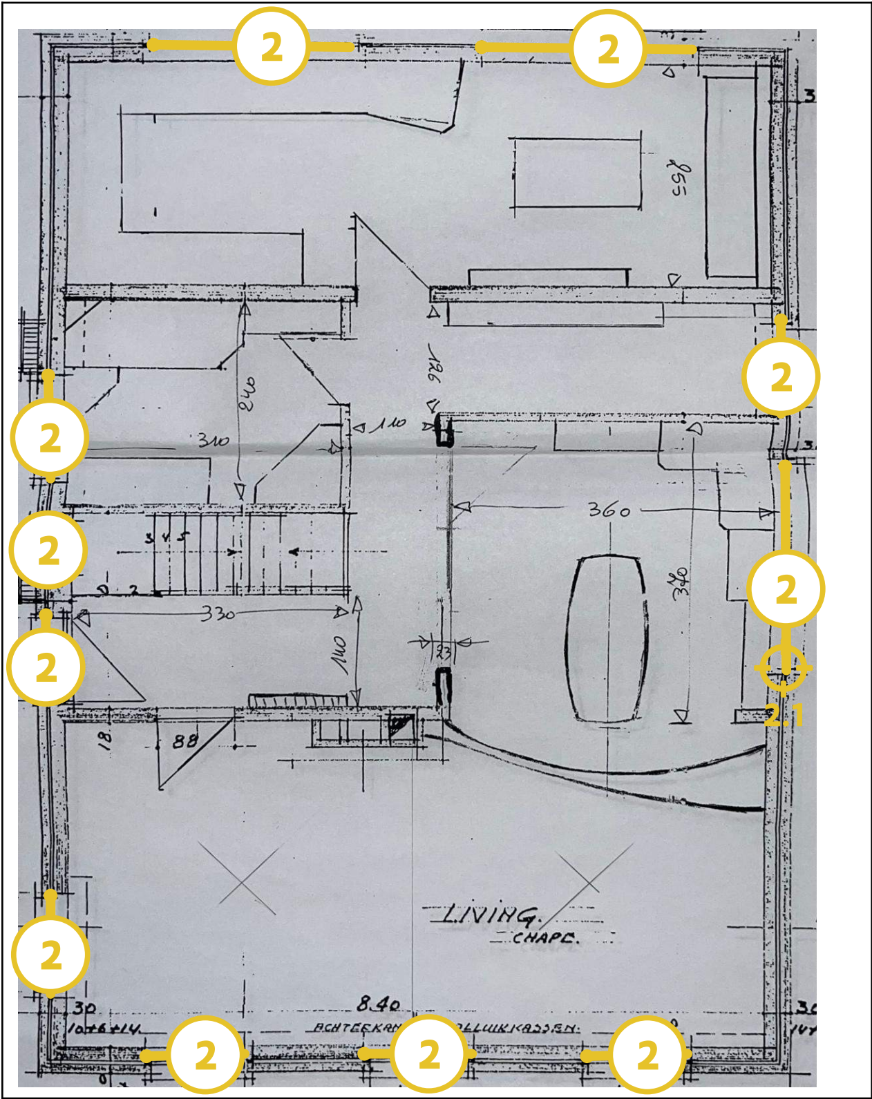
Legende van plan 1.3: Niveau 0 - mastiek
