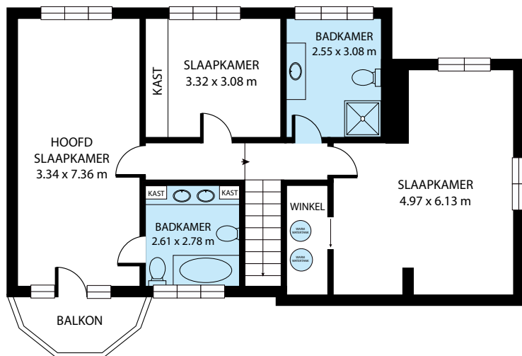
EERSTE VERDIEPING
