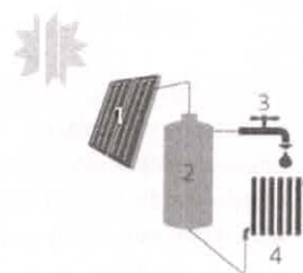
1. Zonnecollector | 2. Opslagvat zonneboiler | 3. Sanitair warm water | 4. Afgifte-element voor ruimteverwarming (opliinnet)
