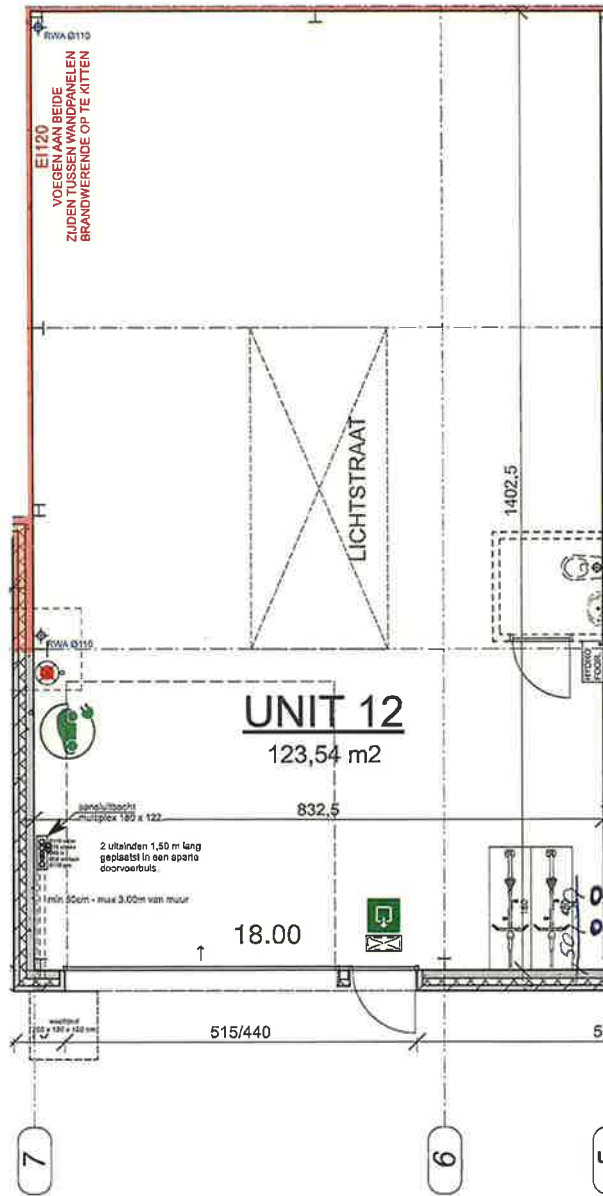
GRONDPLAN // UNIT 12 0m 2m 4m 6m 7m N
