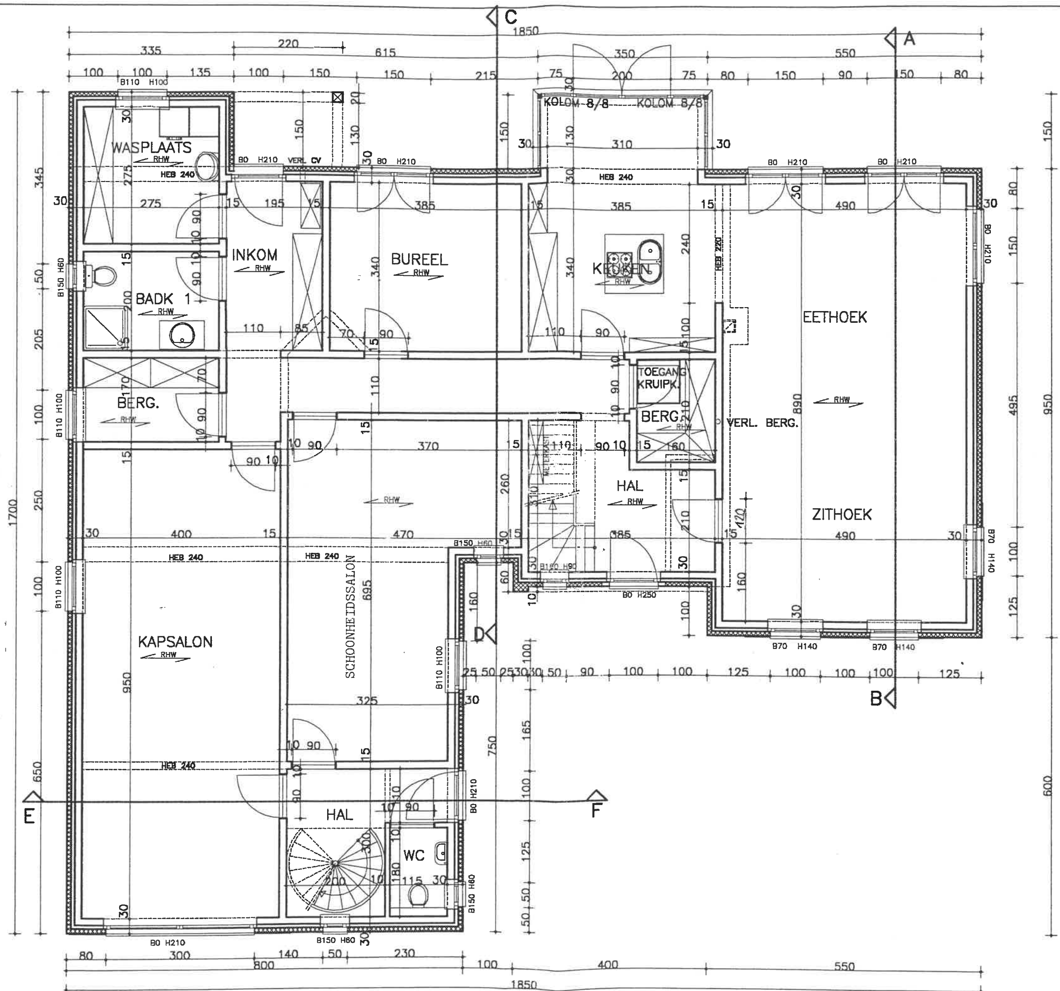
GELIJKVLOERS sch. 1/75
