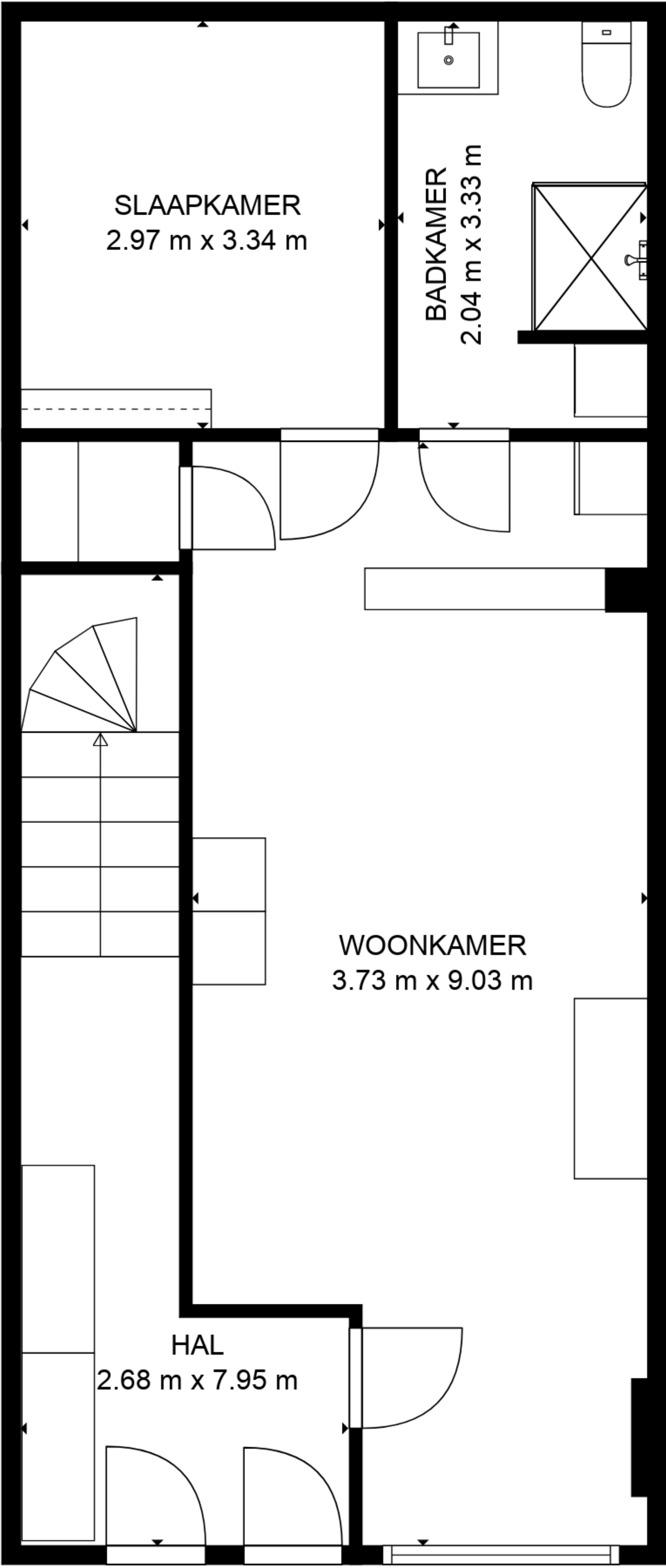
1. GELIJKVLOERS
