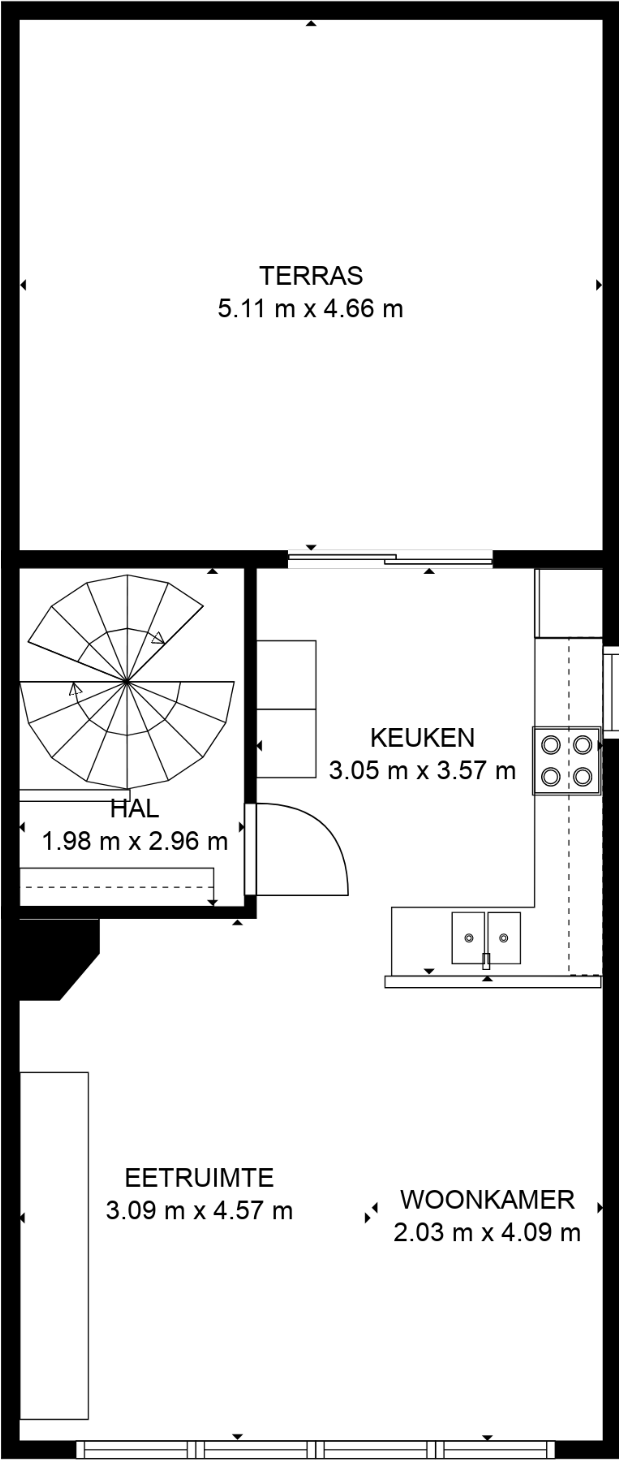
2. EERSTE VERDIEPING
