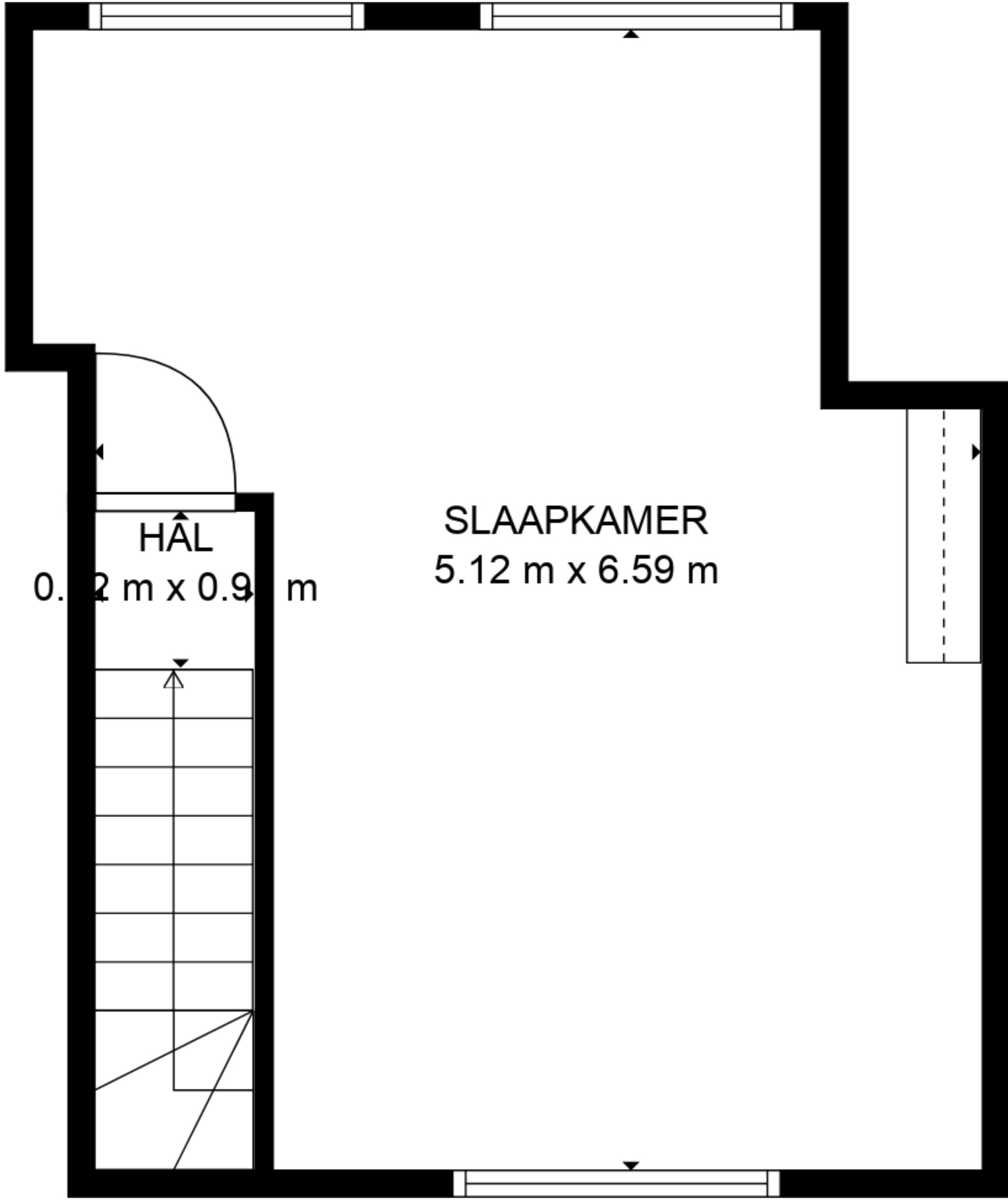
4. DERDE VERDIEPING
