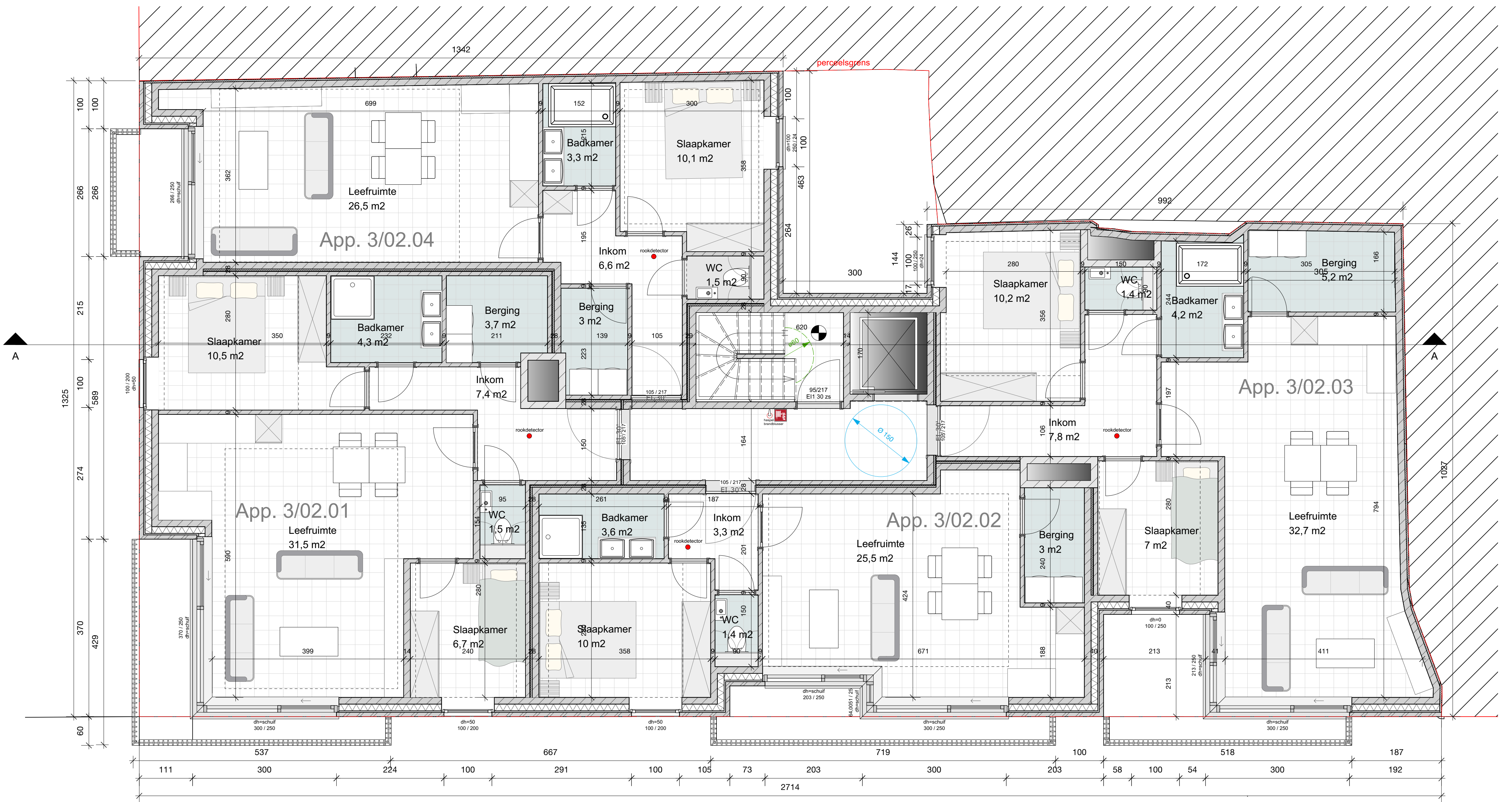
Verdiep +2 1:50
