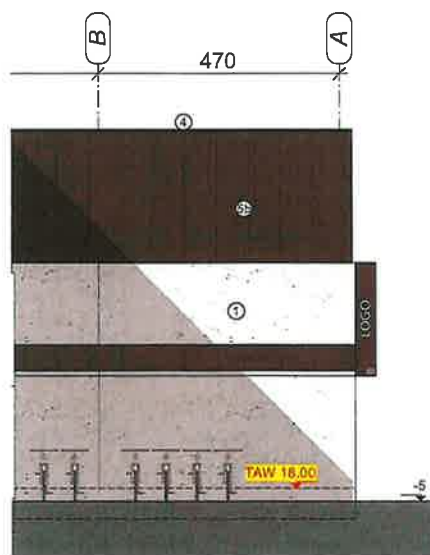
LINKER ZIJGEVEL // UNIT 12
