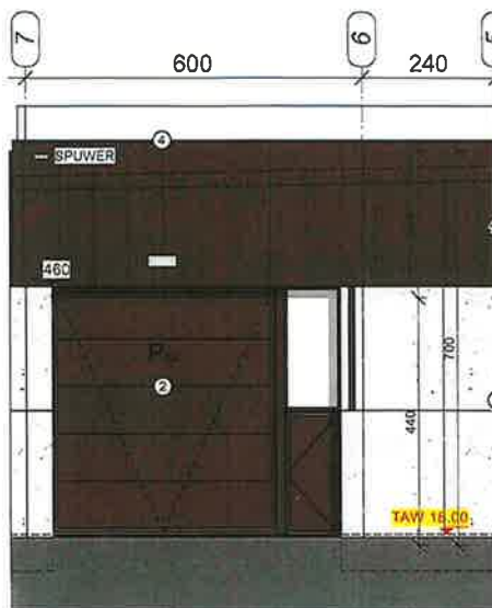
VOORGEVEL // UNIT 12
