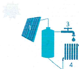
1. Zonnecollector | 2. Opslagvat zonneboiler | 3. Sanitair warm water | 4. Afgeeft element voor ruimteverwarming (radiator)
