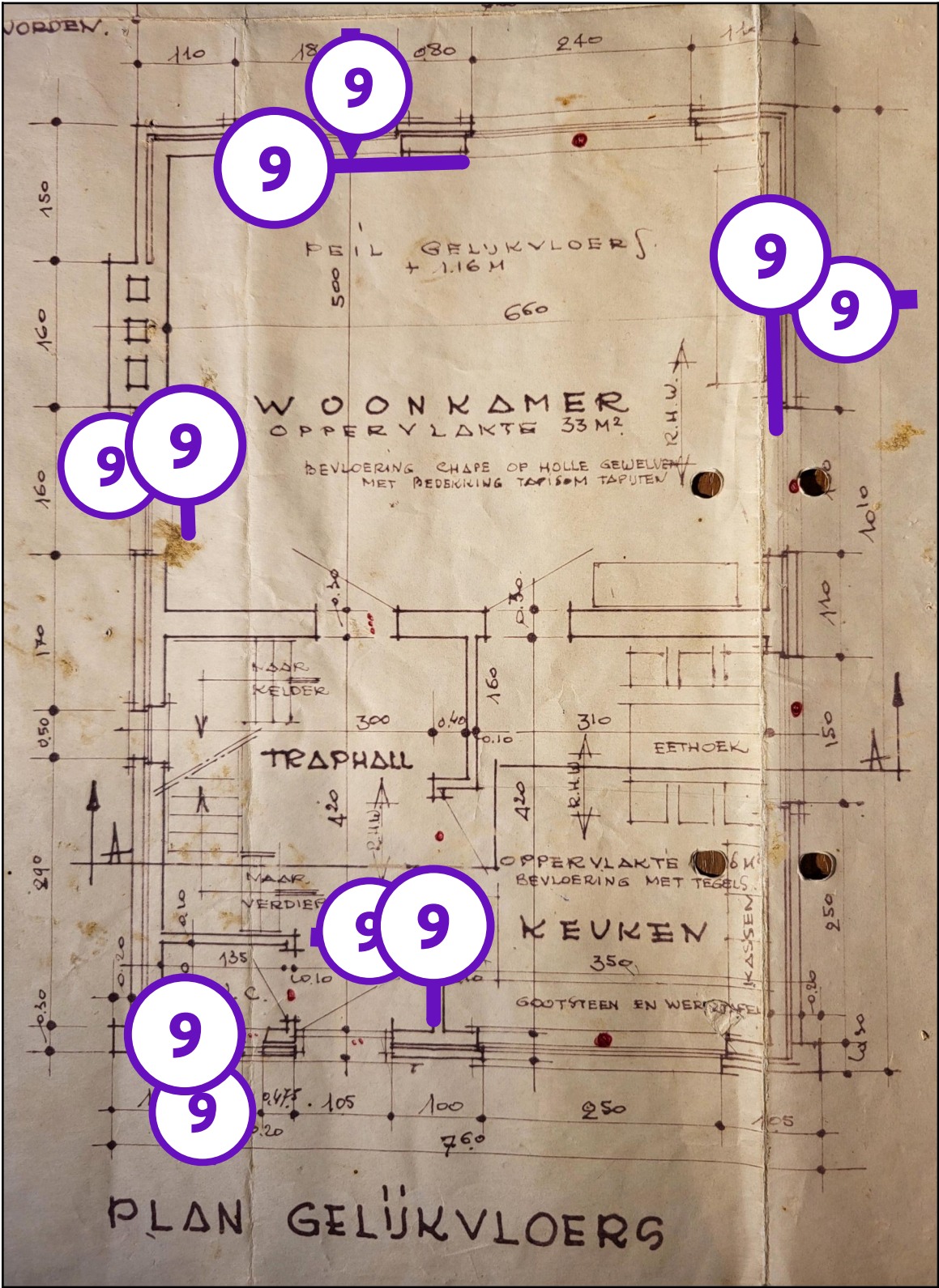
Legende van plan 1.11: Gelijkvloers
