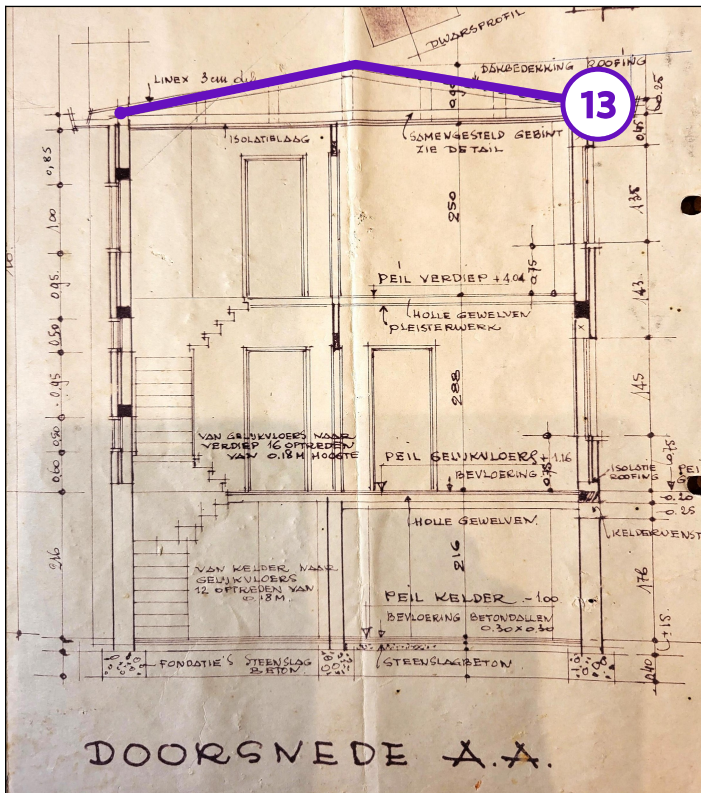
Legende van plan 1.13: Doorsnede
