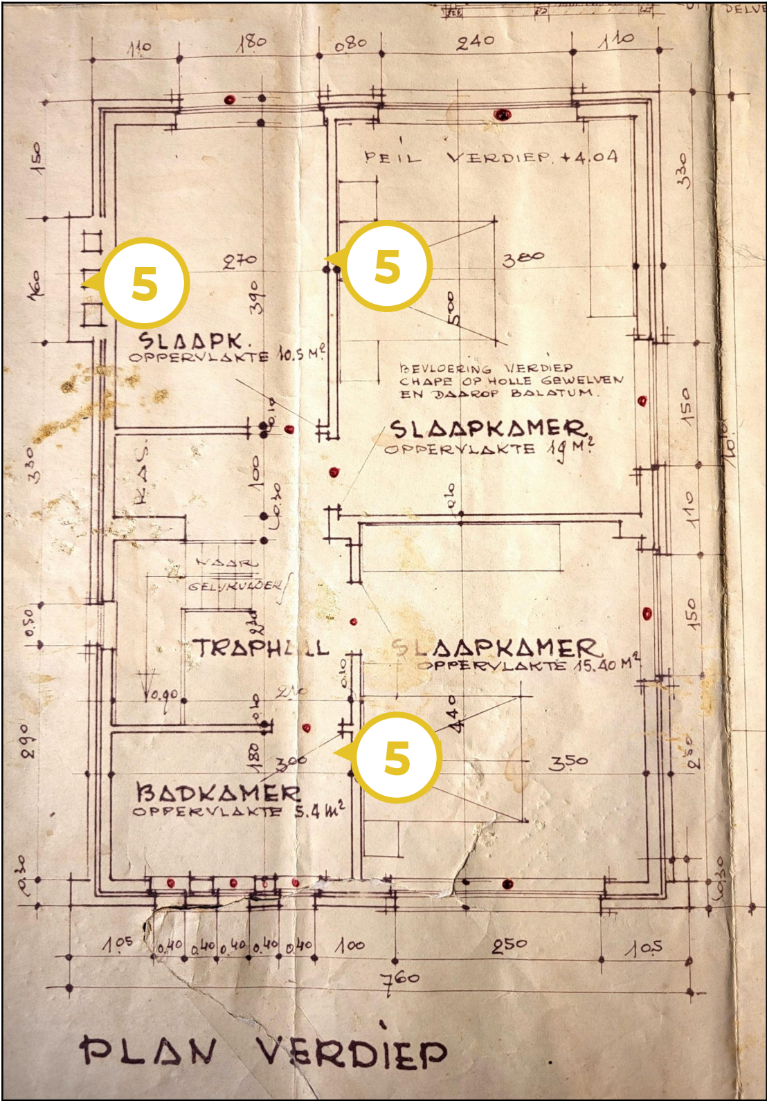
Legende van plan 1.6: Verdieping
