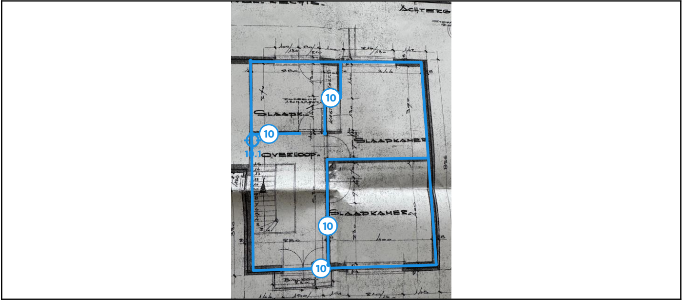
Legende van plan 1.3: Hoofdgebouw plan V+1 Pleisterwerk muren
