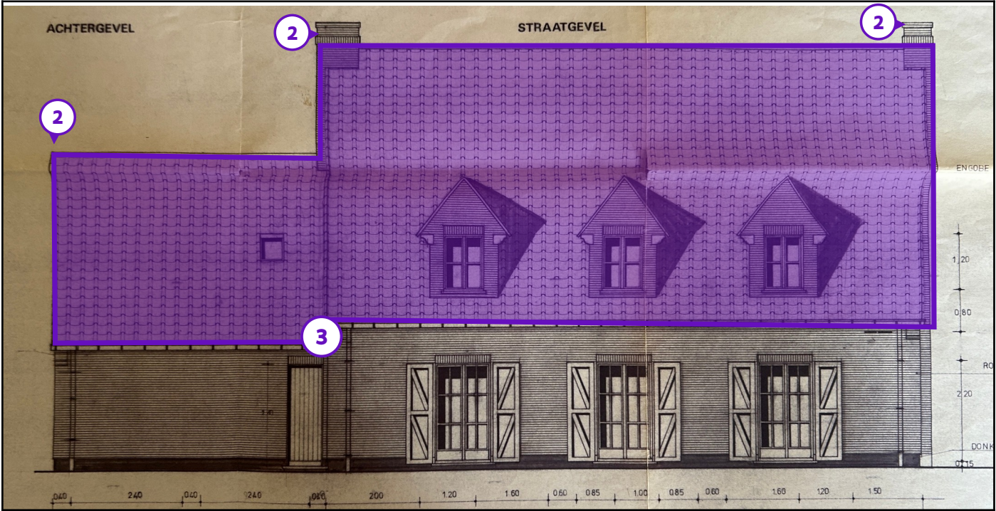
Legende van plan 1.8: dakconstructie
