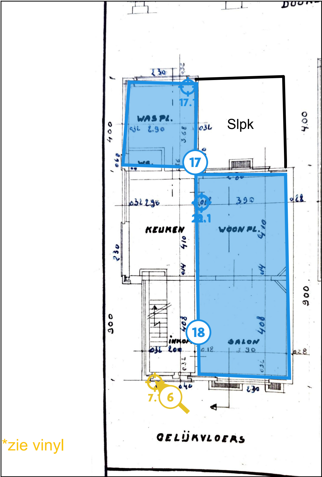
Legende van plan 1.2: GLV
