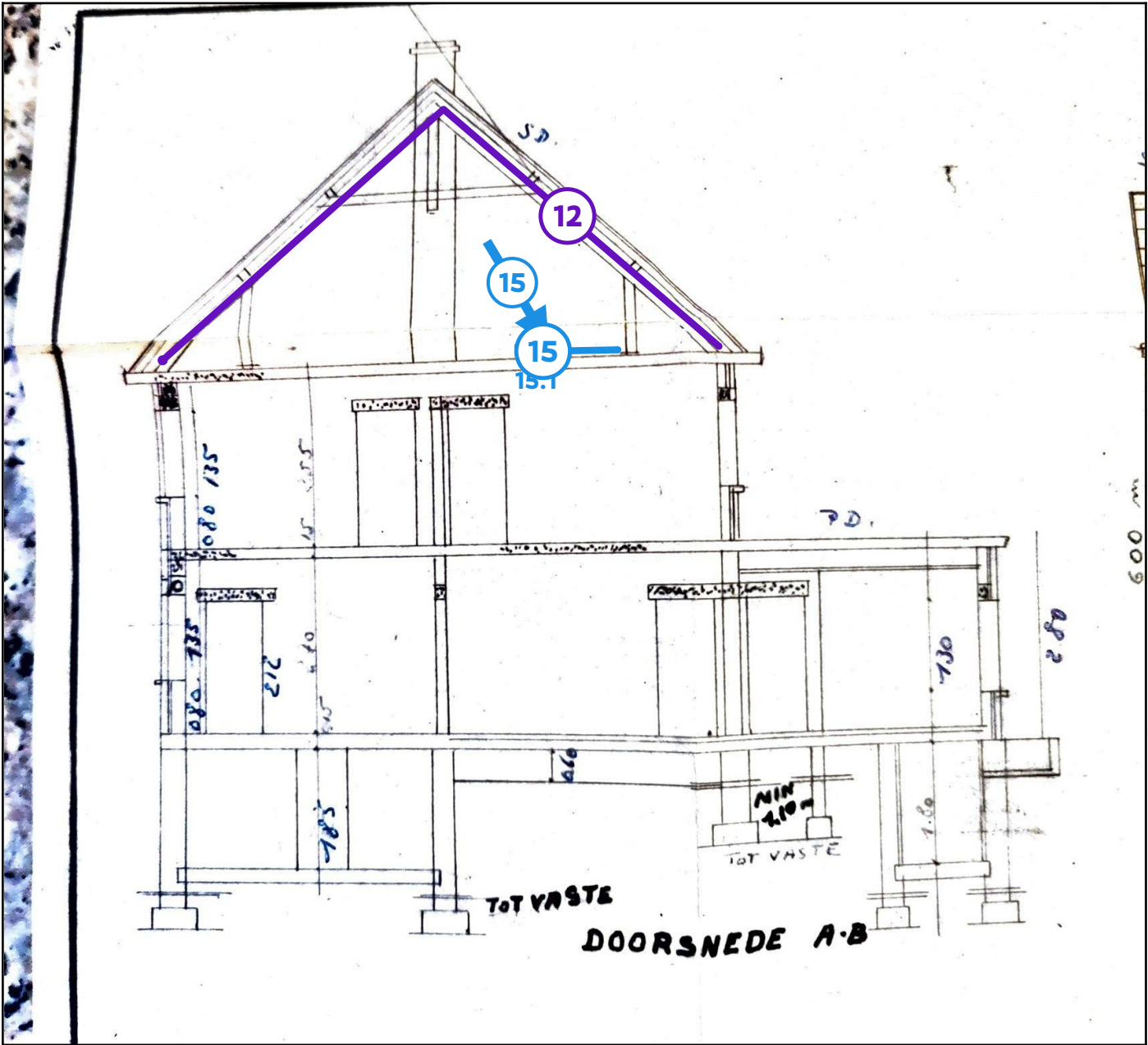
Legende van plan 1.7: Doorsnede
