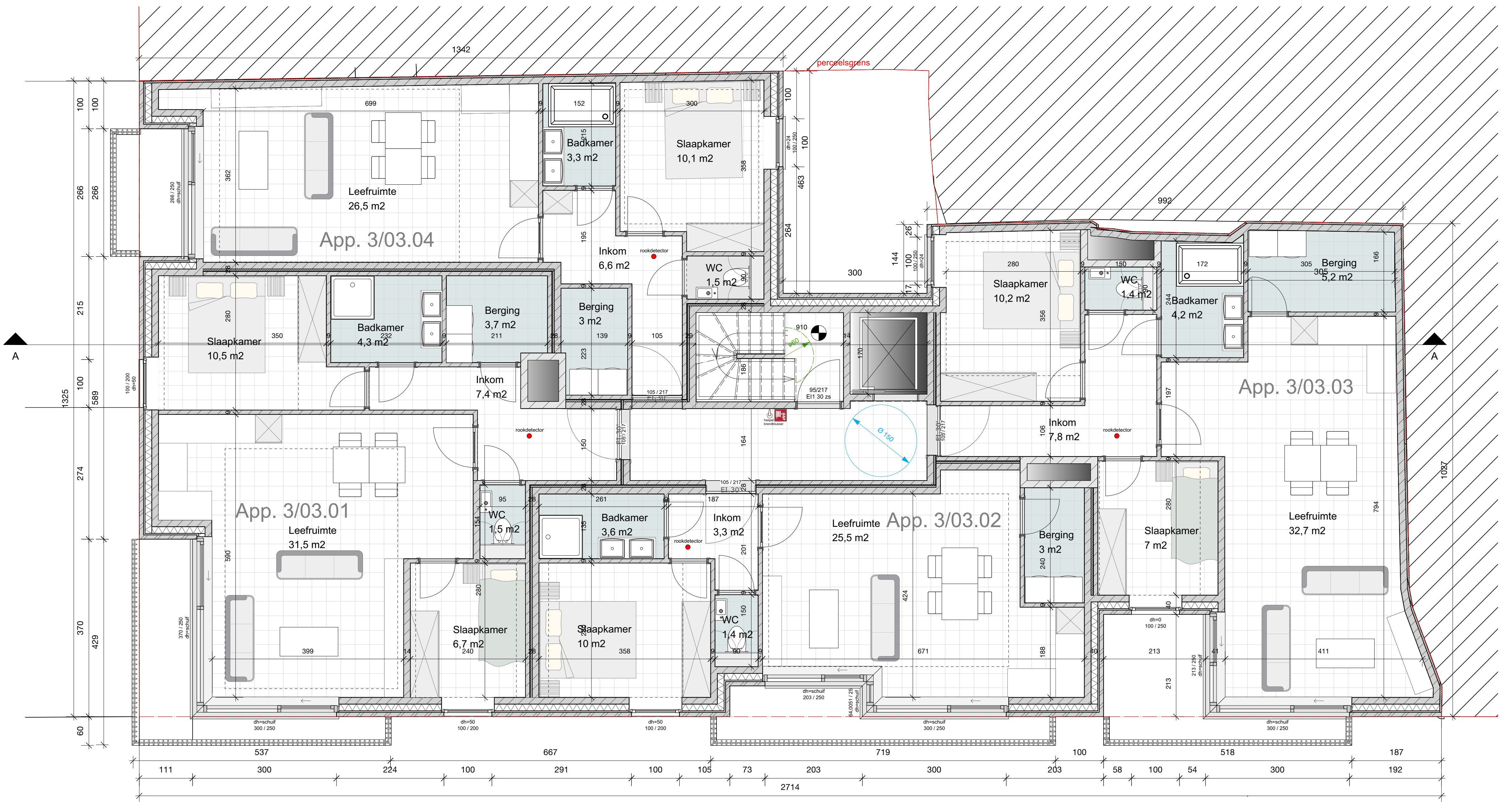
Verdiep +3 1:50
