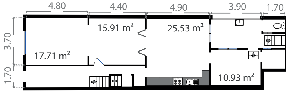
Begane grond
