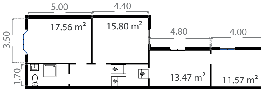
1e Verdieping
