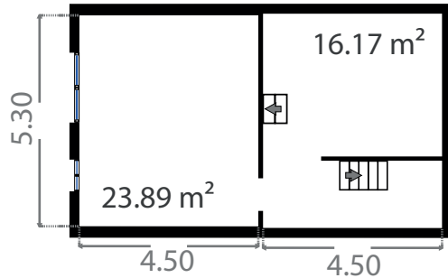
2e Verdieping
