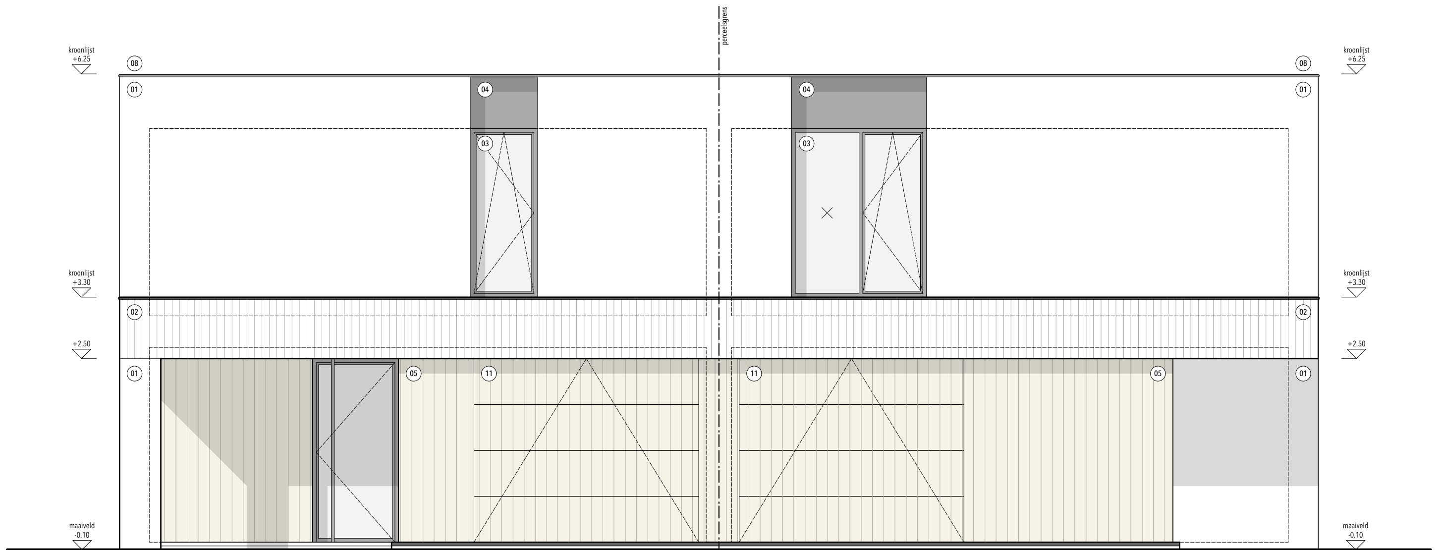
VOORGEVEL SCHAAL 1:50
