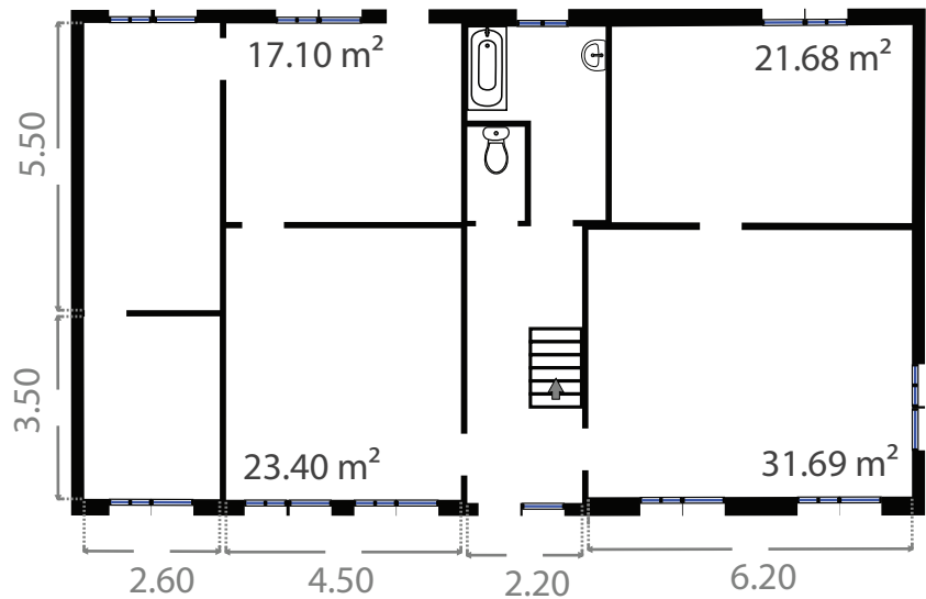
Begane Grond
