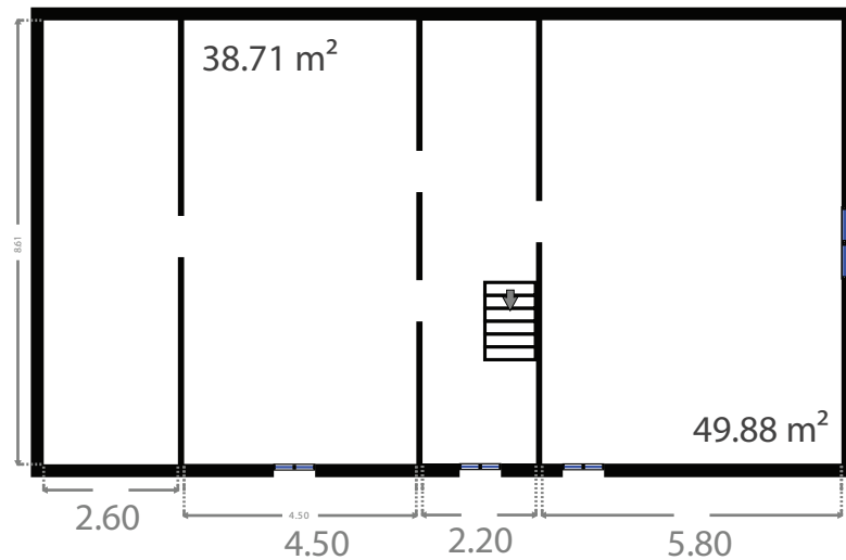
1e verdiep
