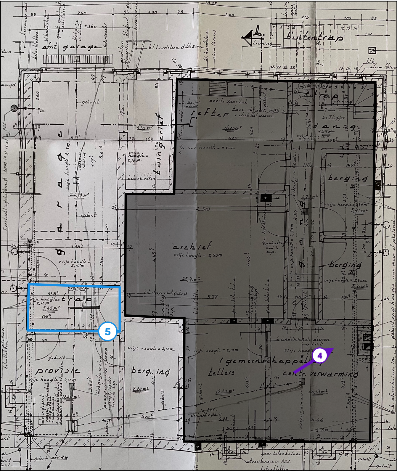
Legende van plan 1.8: Kelder - pleisterwerk wanden
