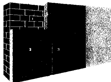
1. Bultengevel | 2. Isolatie | 3. Dampschermbekleding | 4. Binnenafwerking | 5. Stijl- en regelwerk (optioneel)
