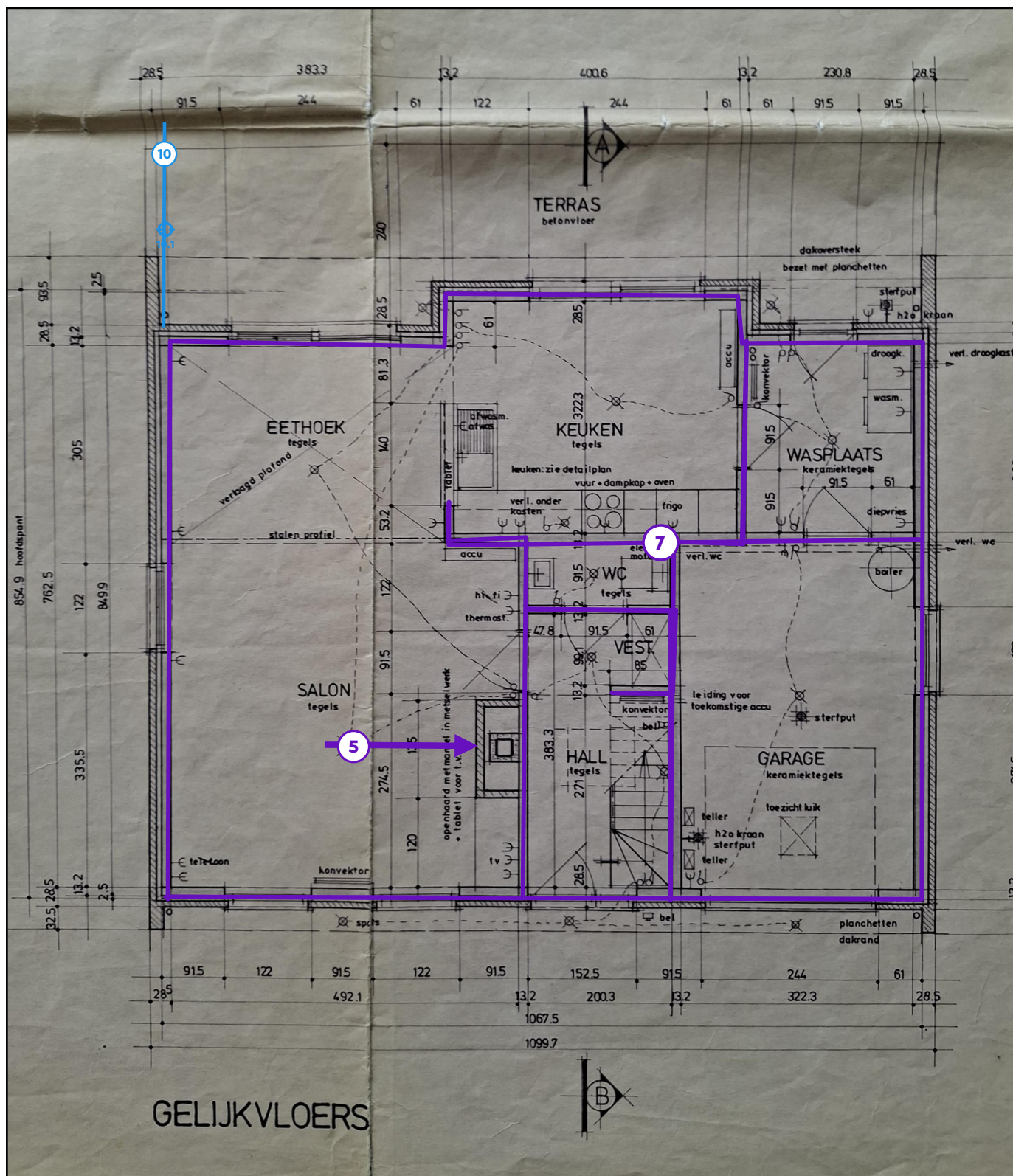
Legende van plan 1.6: Grondplan gelijkvloers
