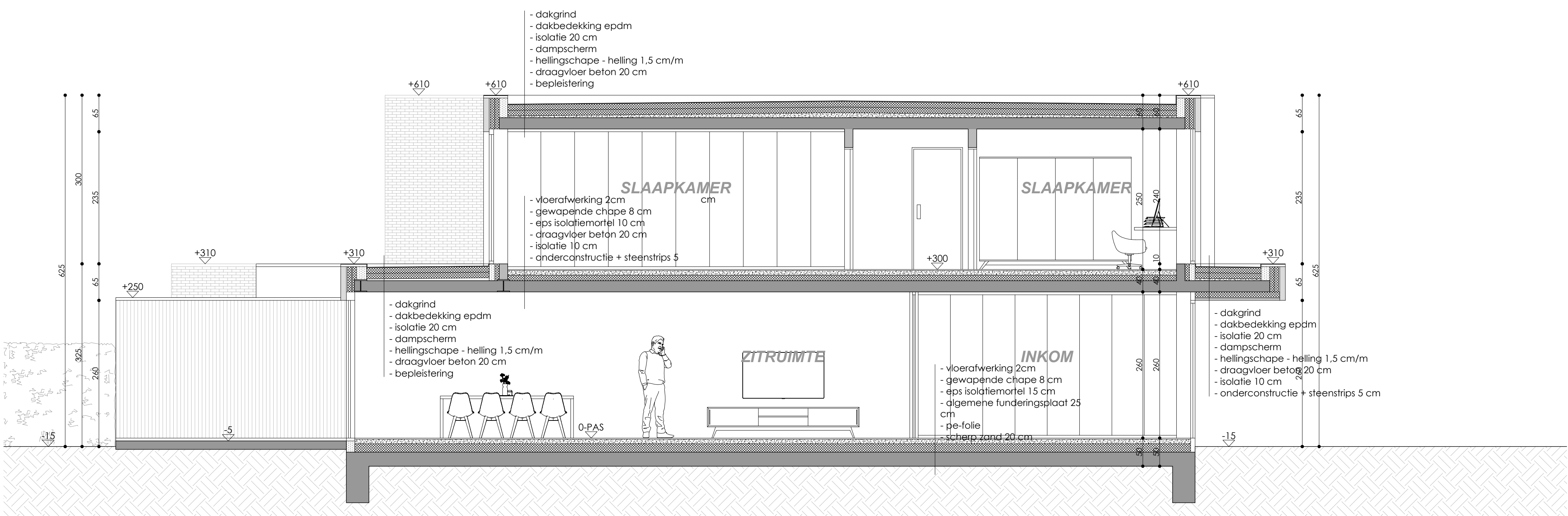
SNEDE CC'
