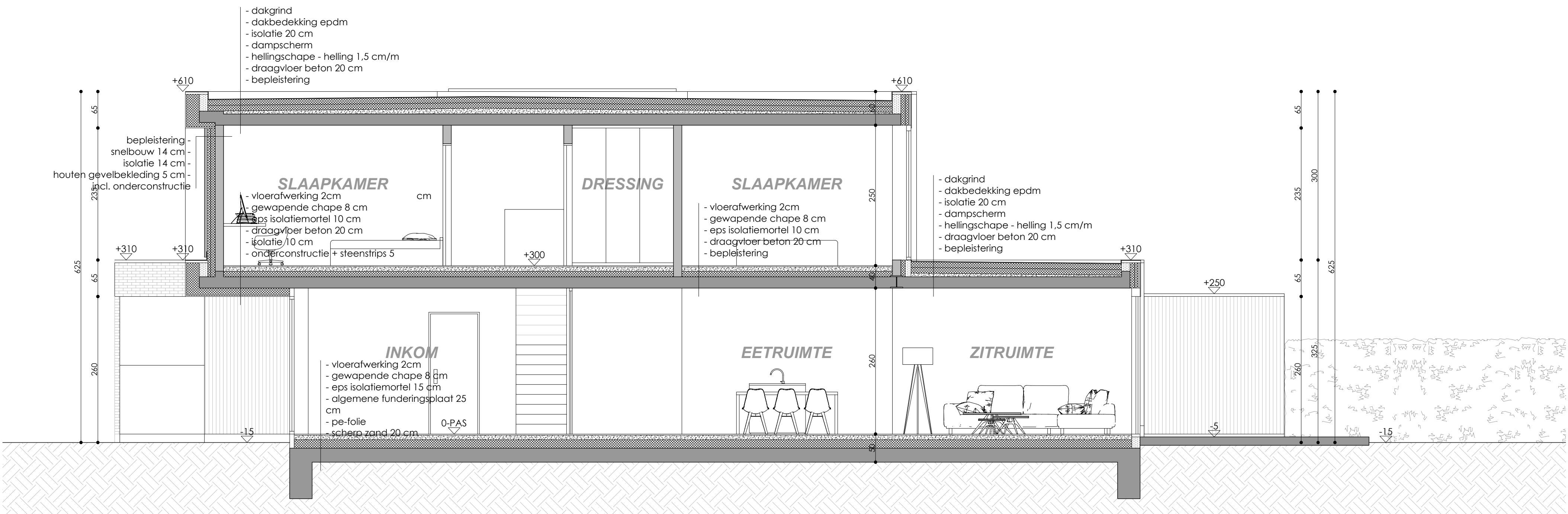
SNEDE BB'
