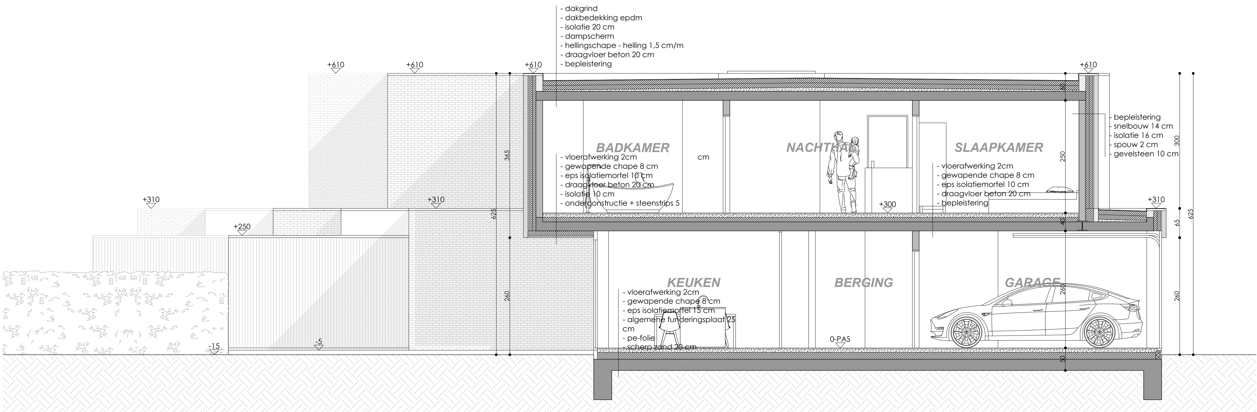
SNEDE AA'
