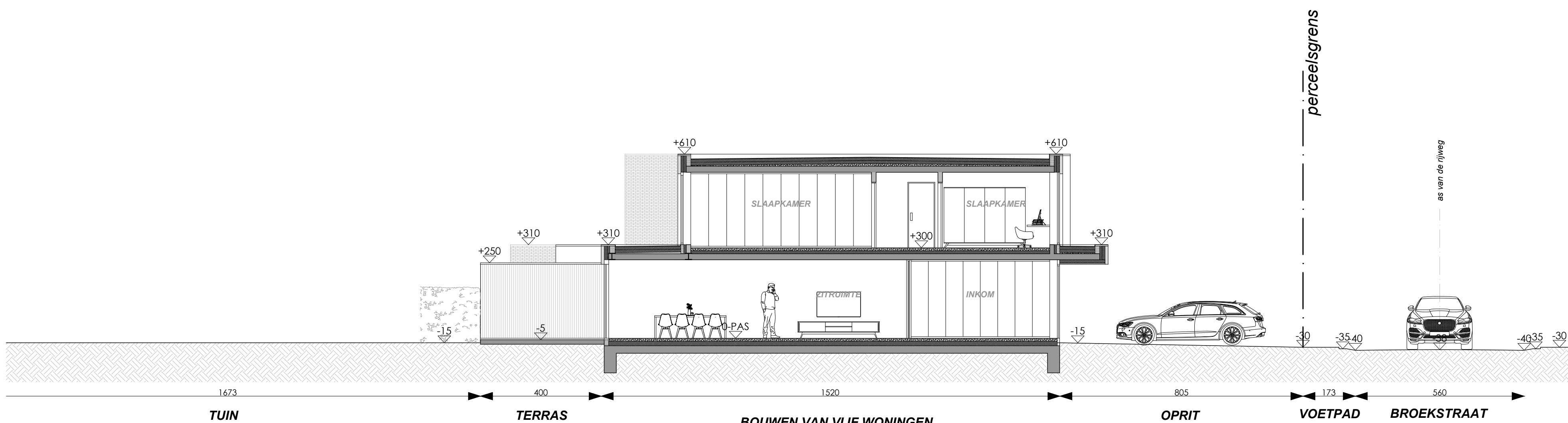
TERREINPROFIEL BB'
