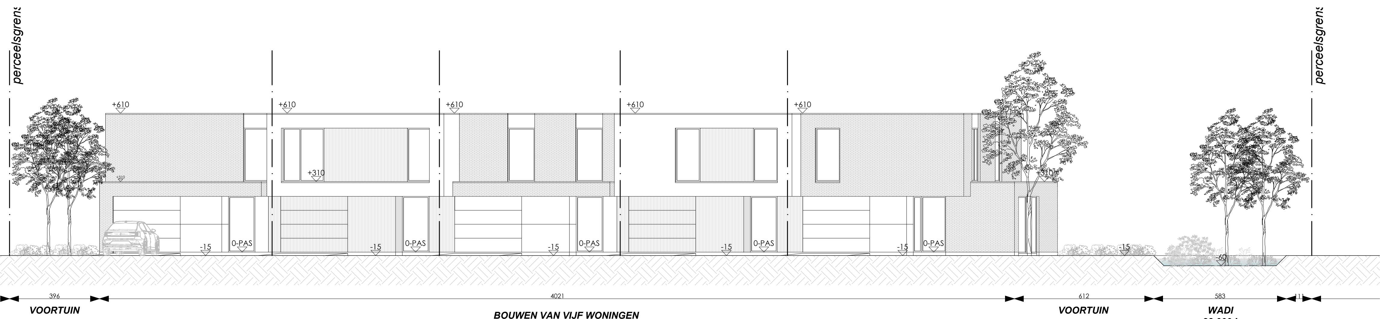
TERREINPROFIEL AA'
