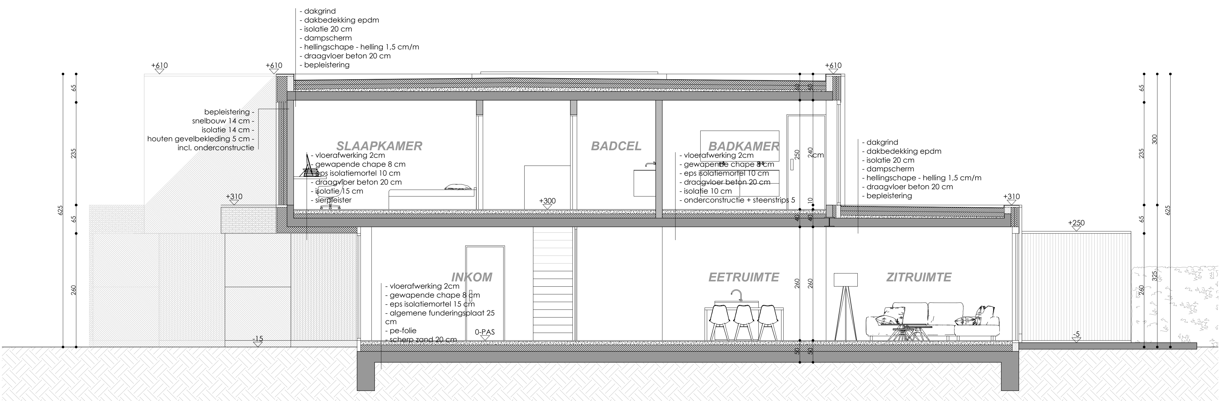
SNEDE DD'
