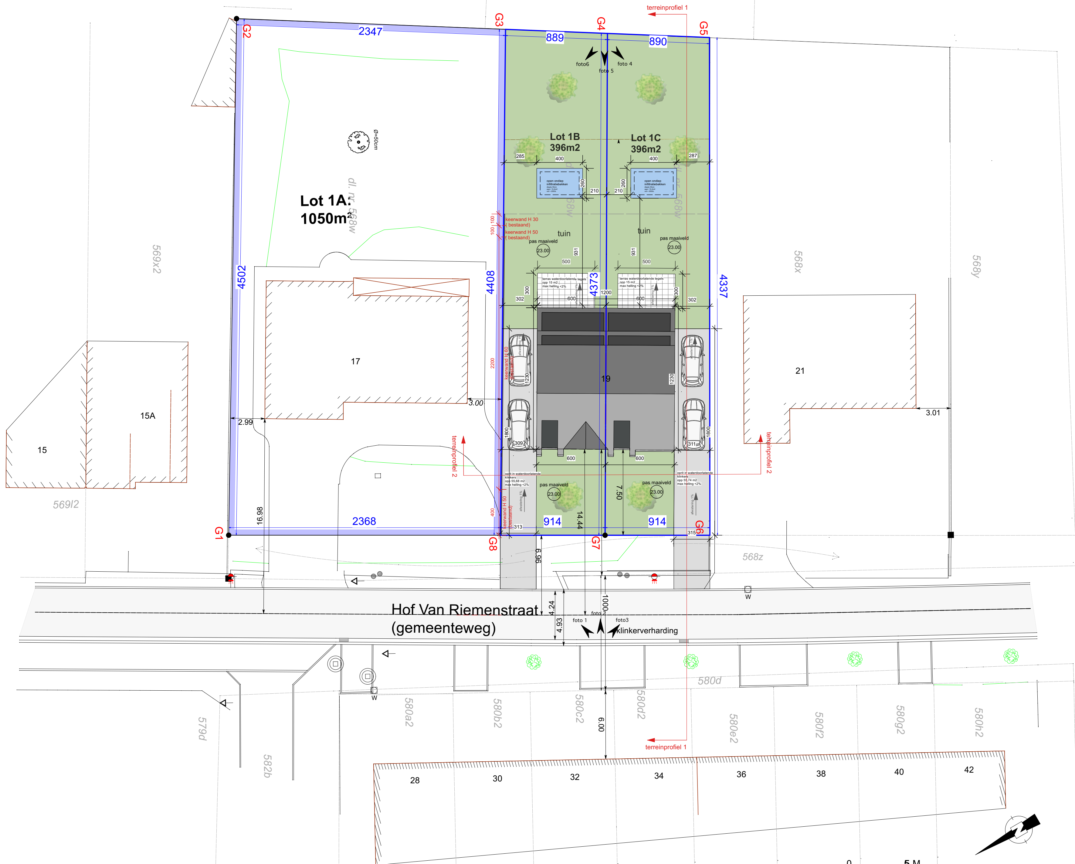
Inplantingsplan nieuwe toestand schaal 1/200
