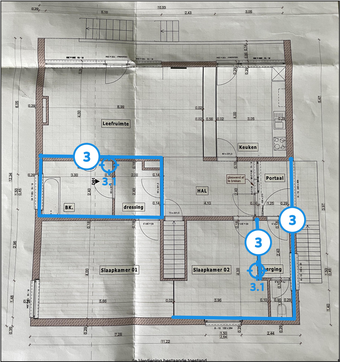
Legende van plan 1.6: grondplan verdiep 1
