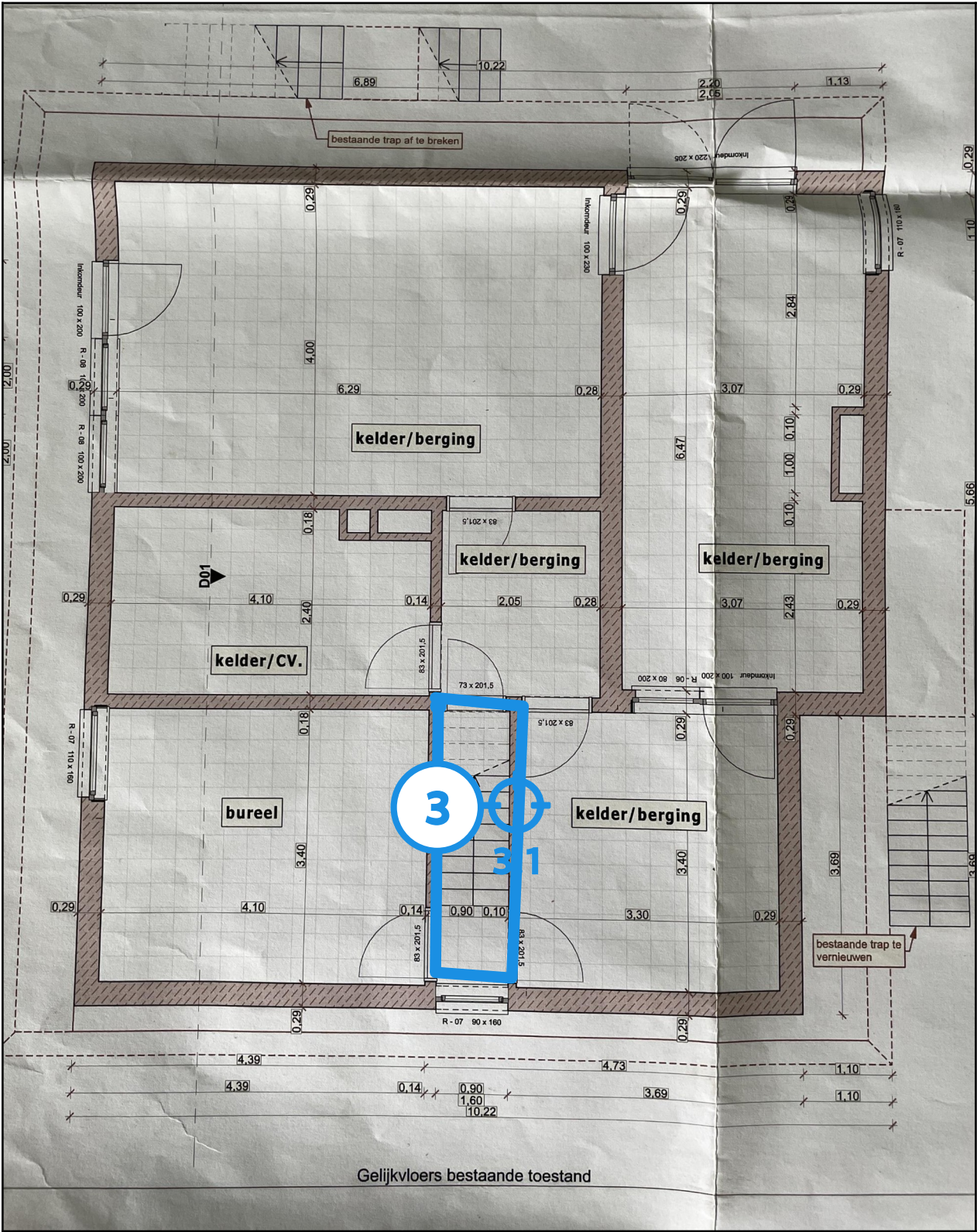
Legende van plan 1.3: grondplan kelder
