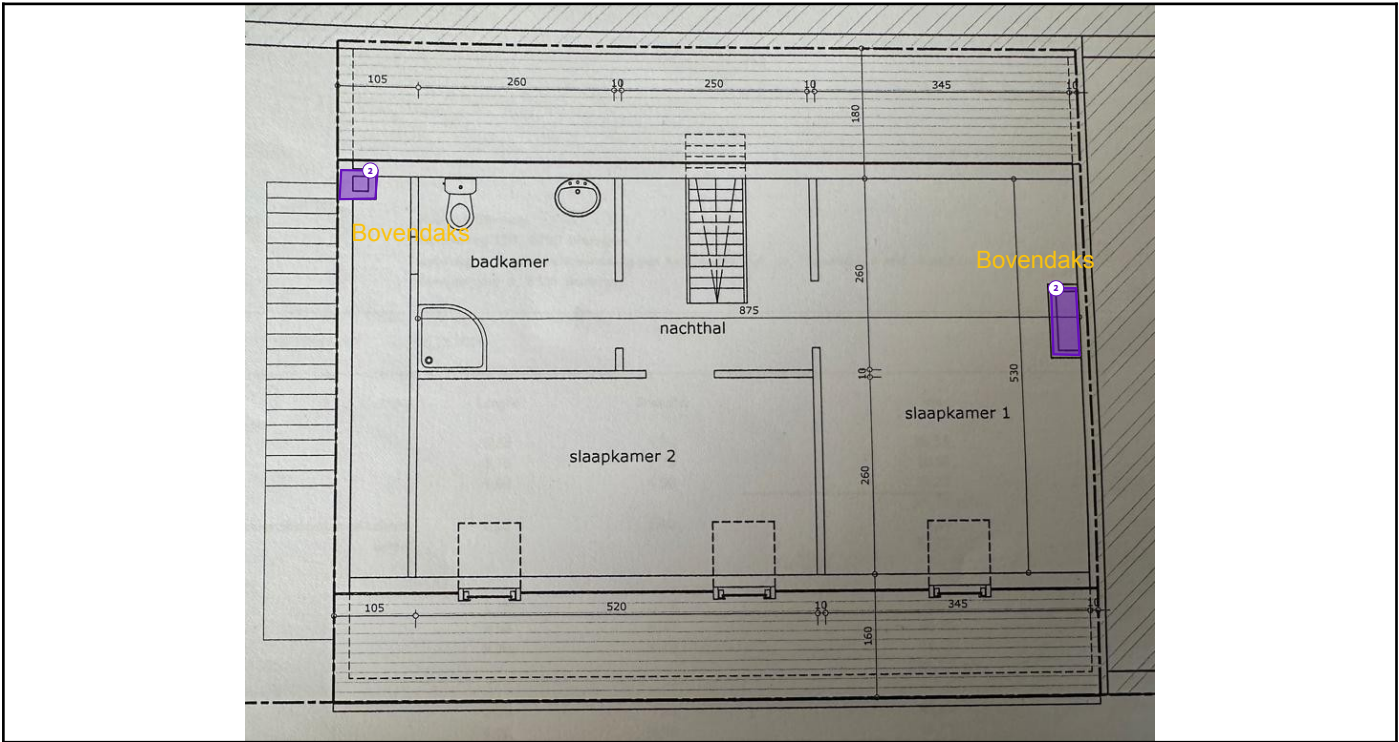
Legende van plan 1.3: Grondplan zolderverdieping (schoorstenen)
