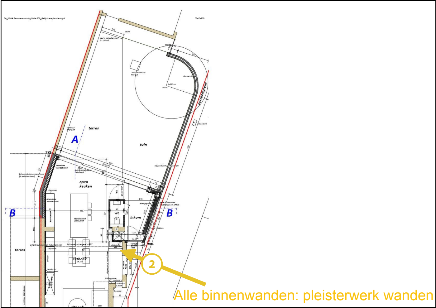
Legende van plan 1.4: Gelijkvloers deel 2 - pleisterwerk wanden
