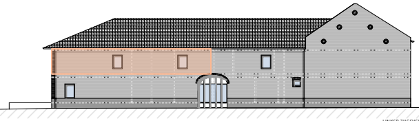
LINKER ZIJGEVEL
