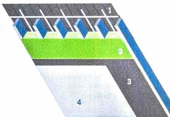
1. Onderdak | 2. Isolatie | 3. Dampscherm | 4. binnenafwerking
