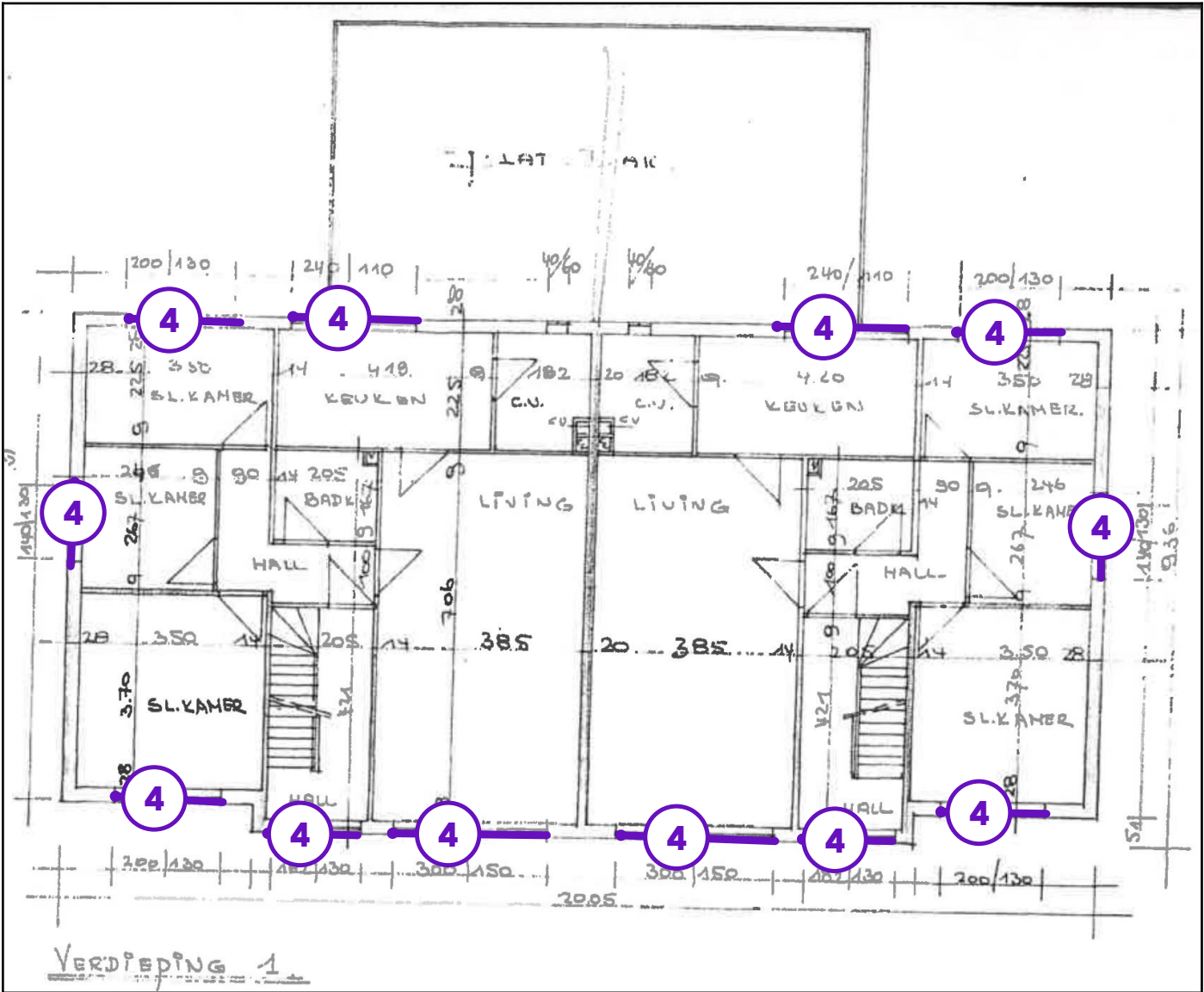
Legende van plan 1.11: 1ste verdieping
