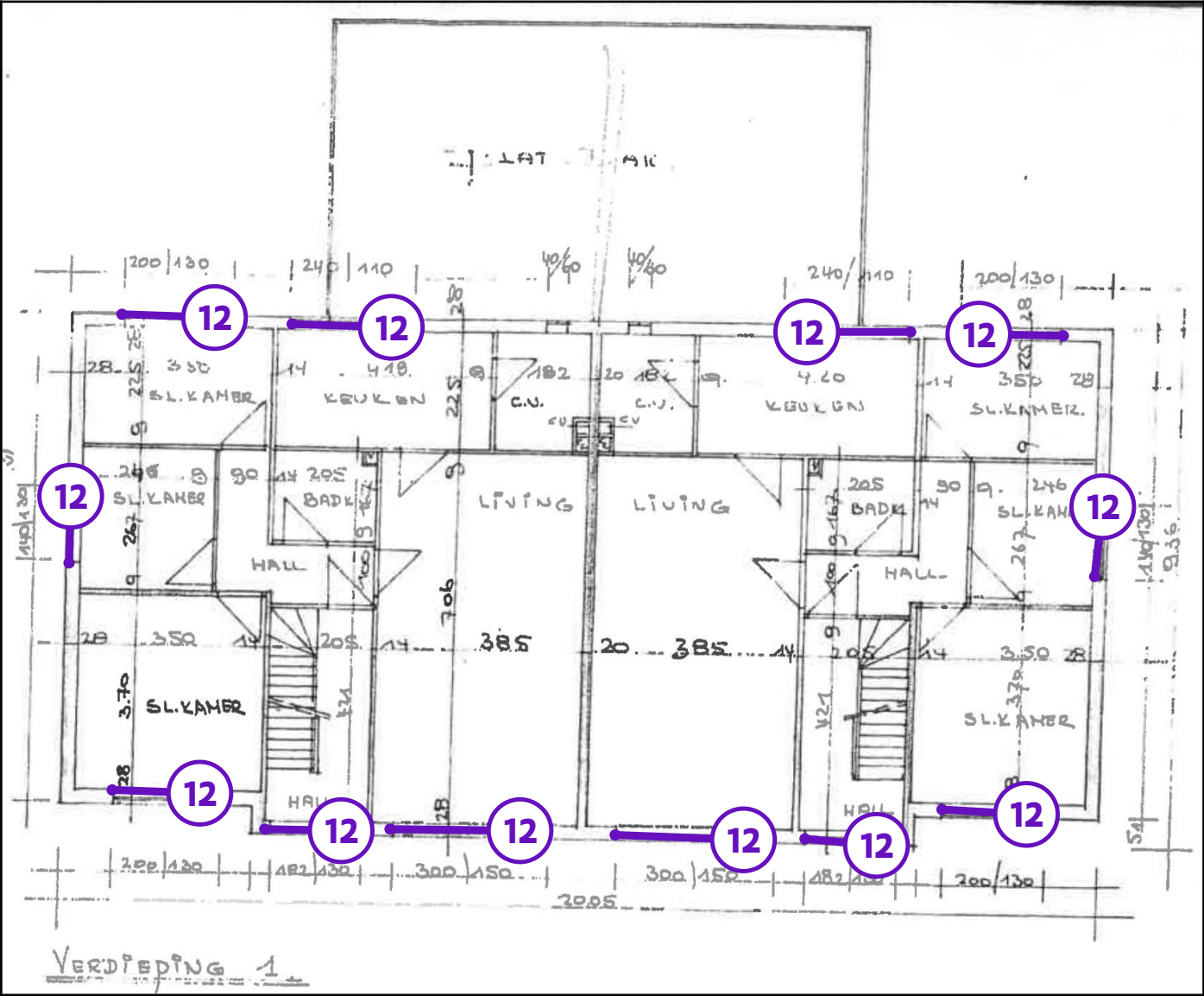
Legende van plan 1.10: 1ste verdieping
