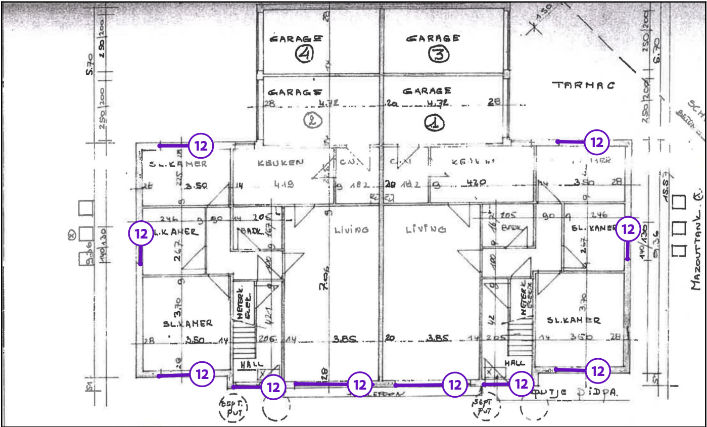
Legende van plan 1.4: plan gelijkvloers
