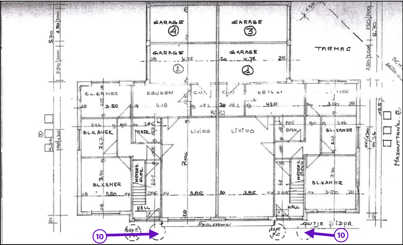
Legende van plan 1.12: plan gelijkvloers
