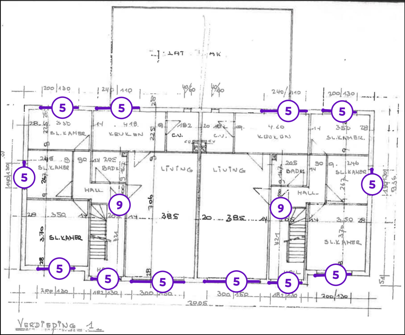
Legende van plan 1.9: 1ste verdieping
