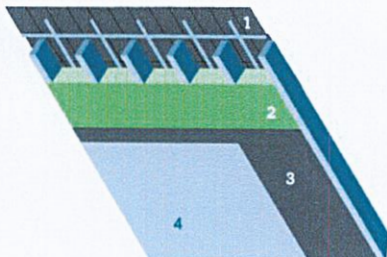
1. Onderdak | 2. Isolatie | 3. Dampscherm | 4. Binnenafwerking
