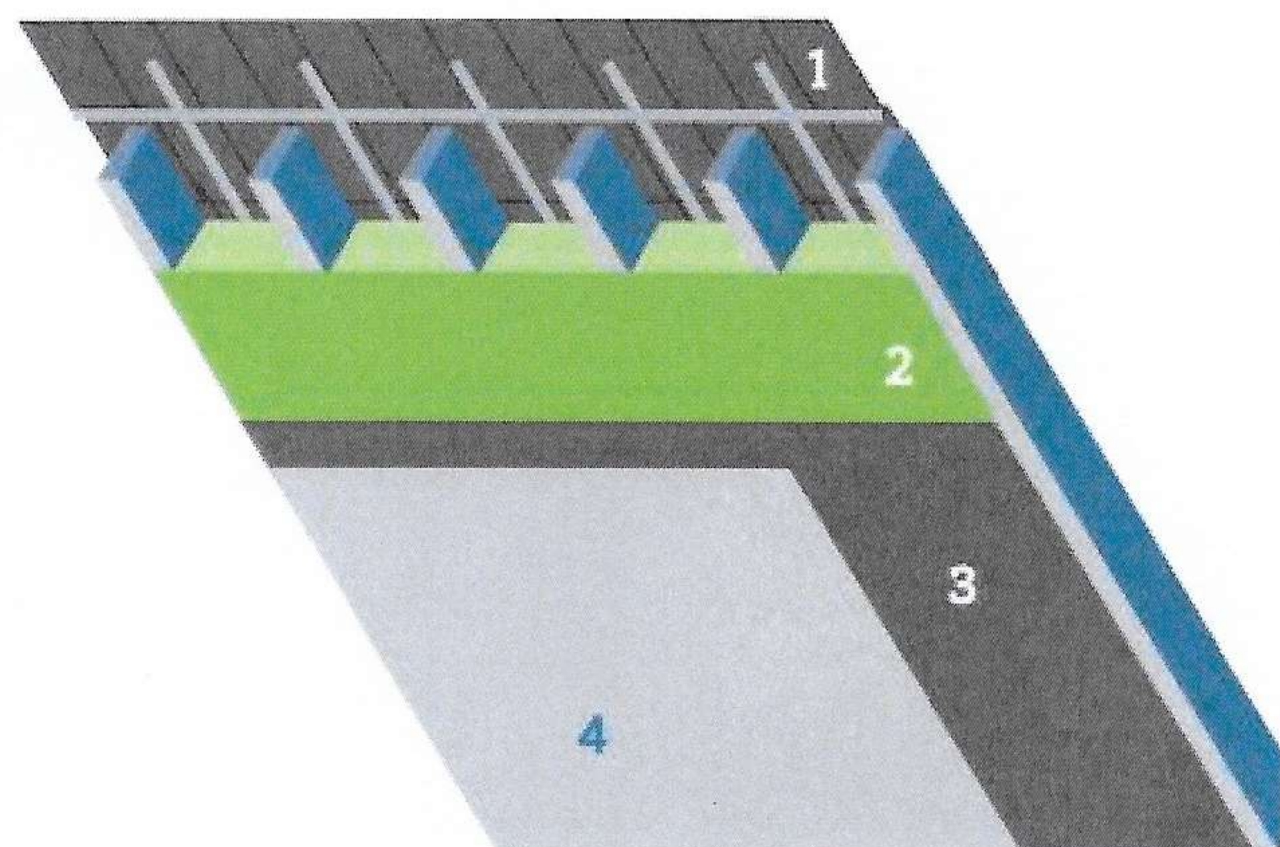
1. Onderdak | 2. Isolatie | 3. Dampscherm | 4. binnenafwerking
