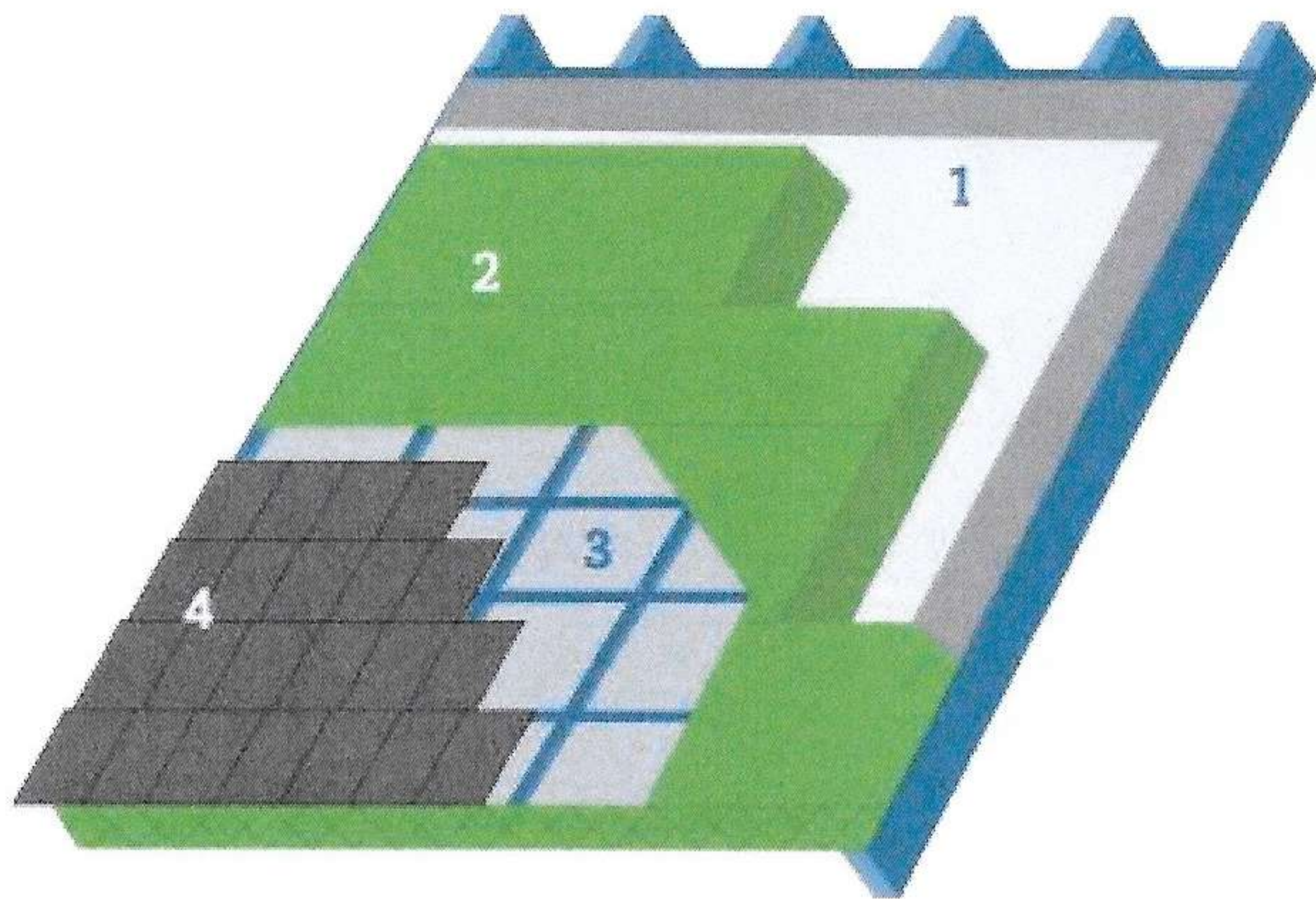
1. Dampscherm | 2. Isolatie | 3. Onderdak | 4. Dakbekleding
