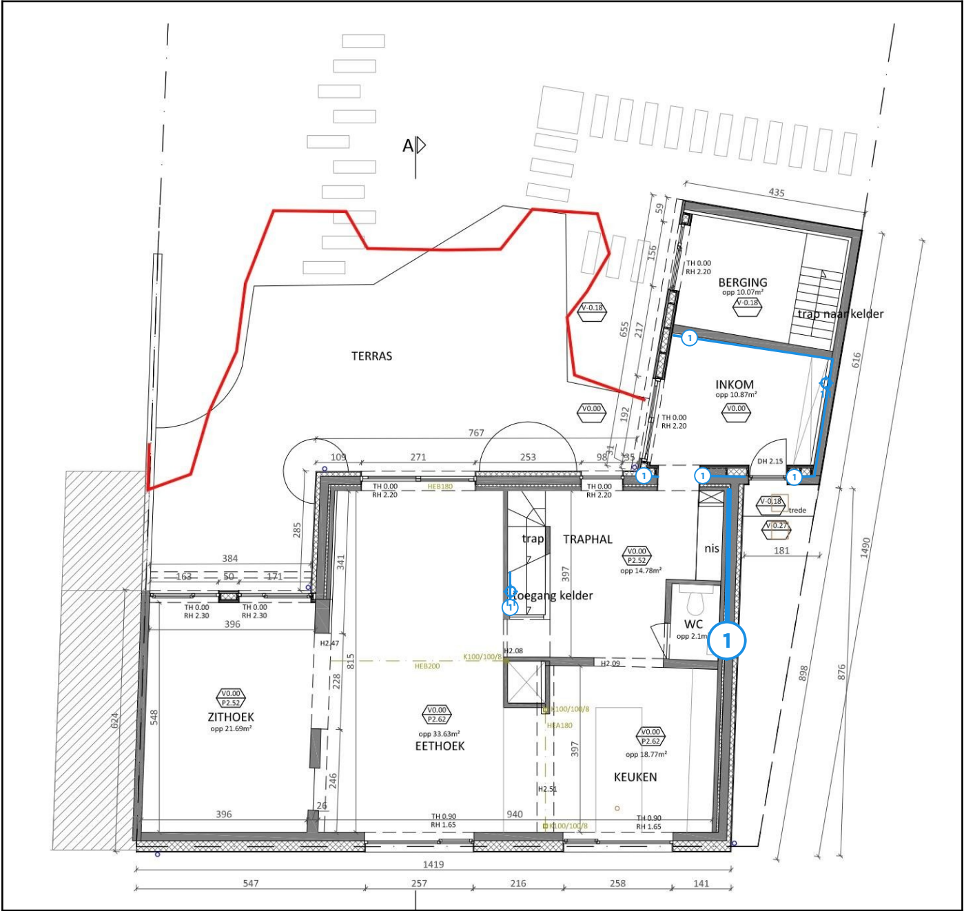
Legende van plan 1.2: Pleisterwerk gelijkvloers
