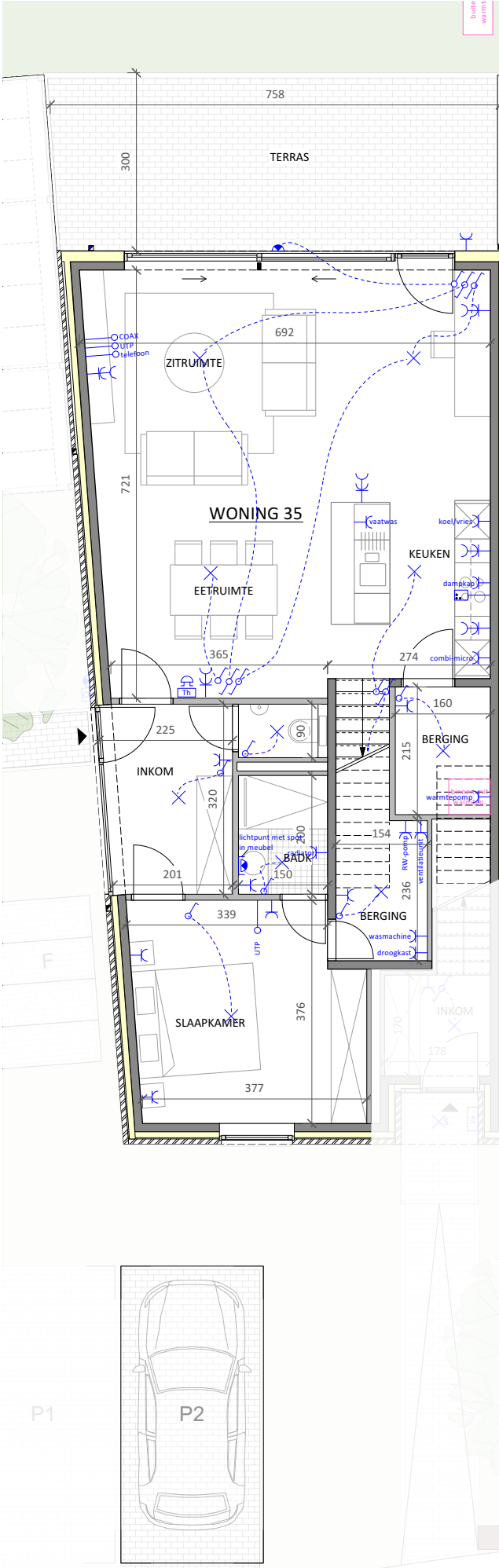
GELIJKVLOERS
