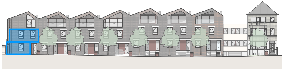
VOORGEVEL
