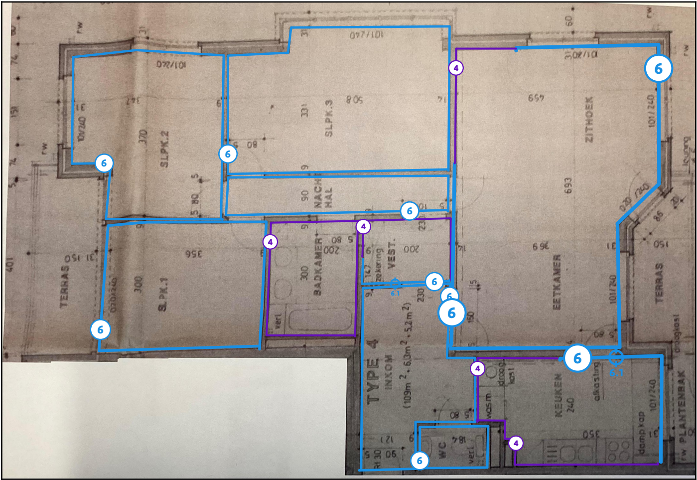
Legende van plan 1.1: Grondplan appartement
