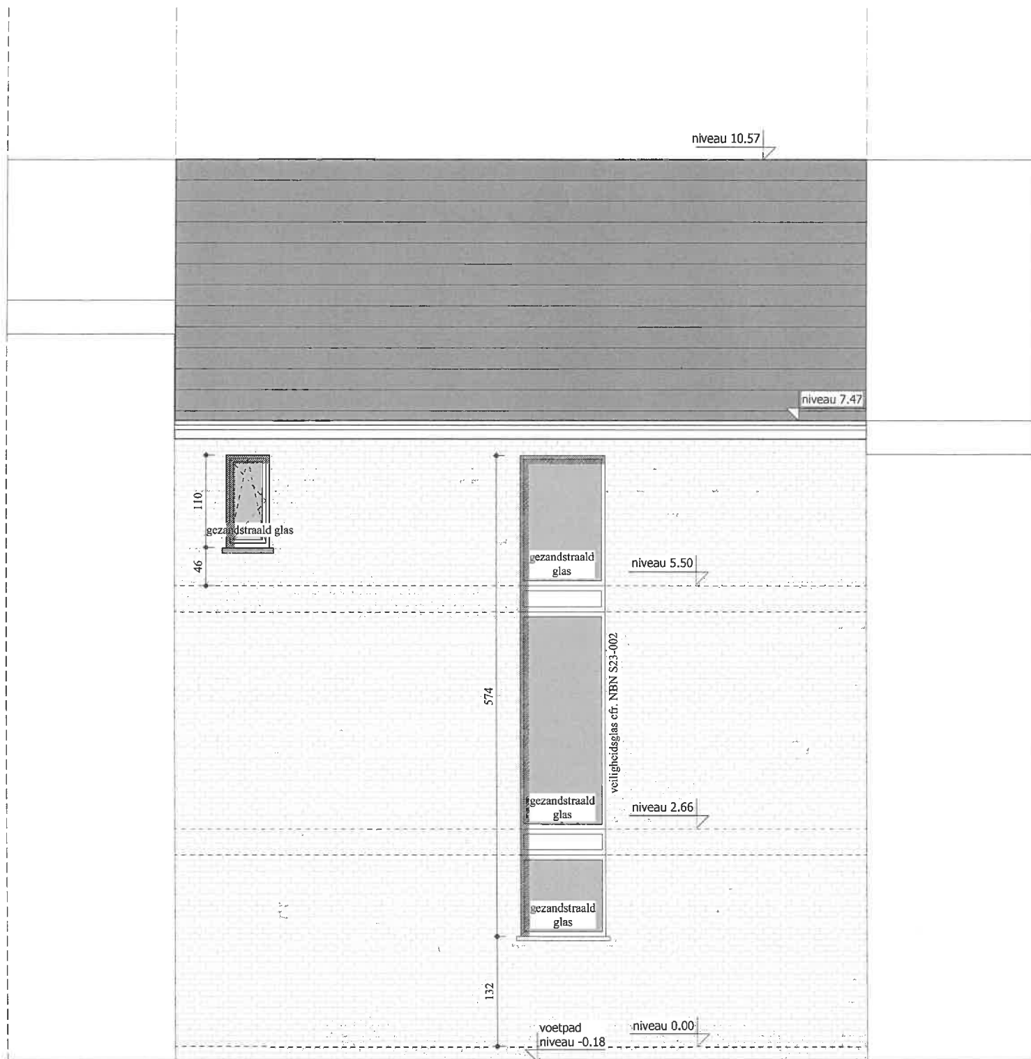
■ ■ ■ ACHTERGEVEL SCH.1/50
