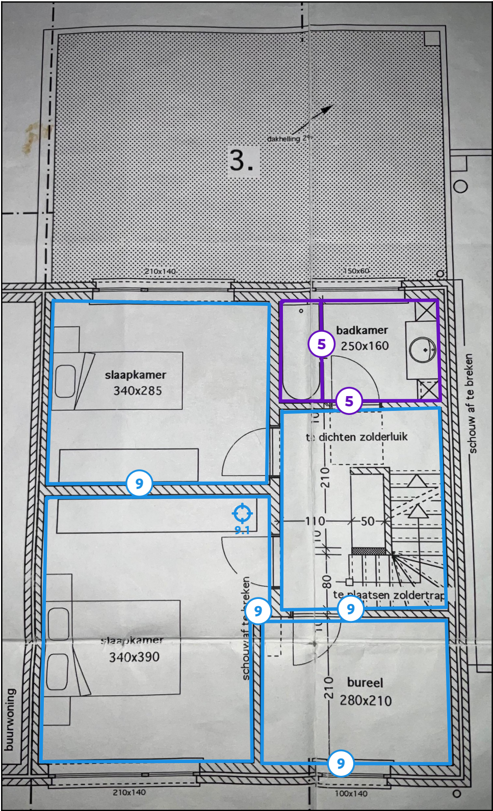
Legende van plan 1.4: Verdiep - pleisterwerk wanden
