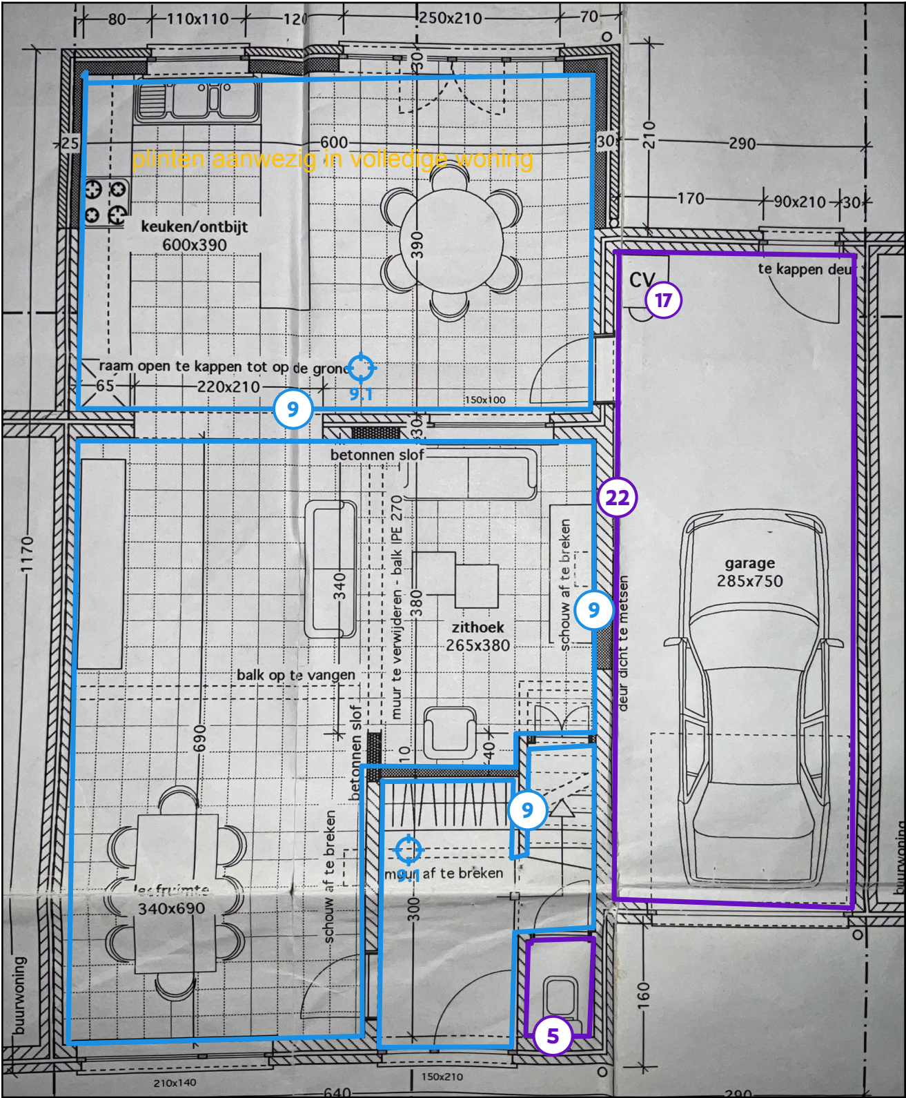
Legende van plan 1.1: Gelijkvloers - pleisterwerk wanden
