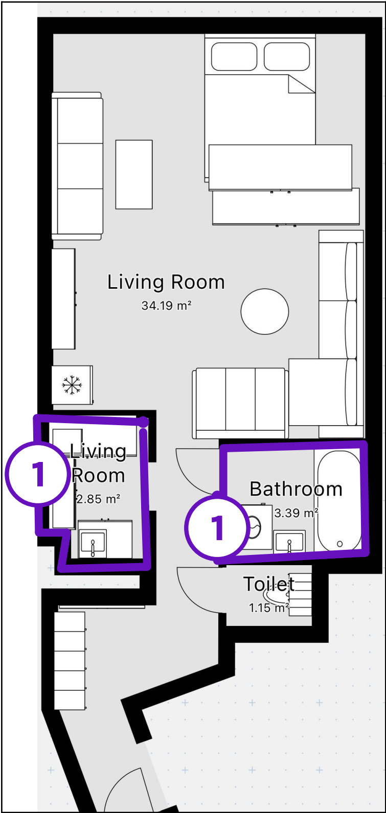
Legende van plan 1.3: Grondplan
