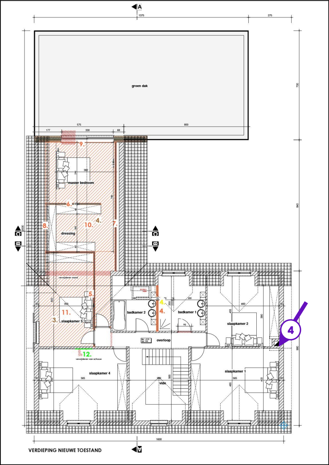
Legende van plan 1.7: afwerking - verdieping
