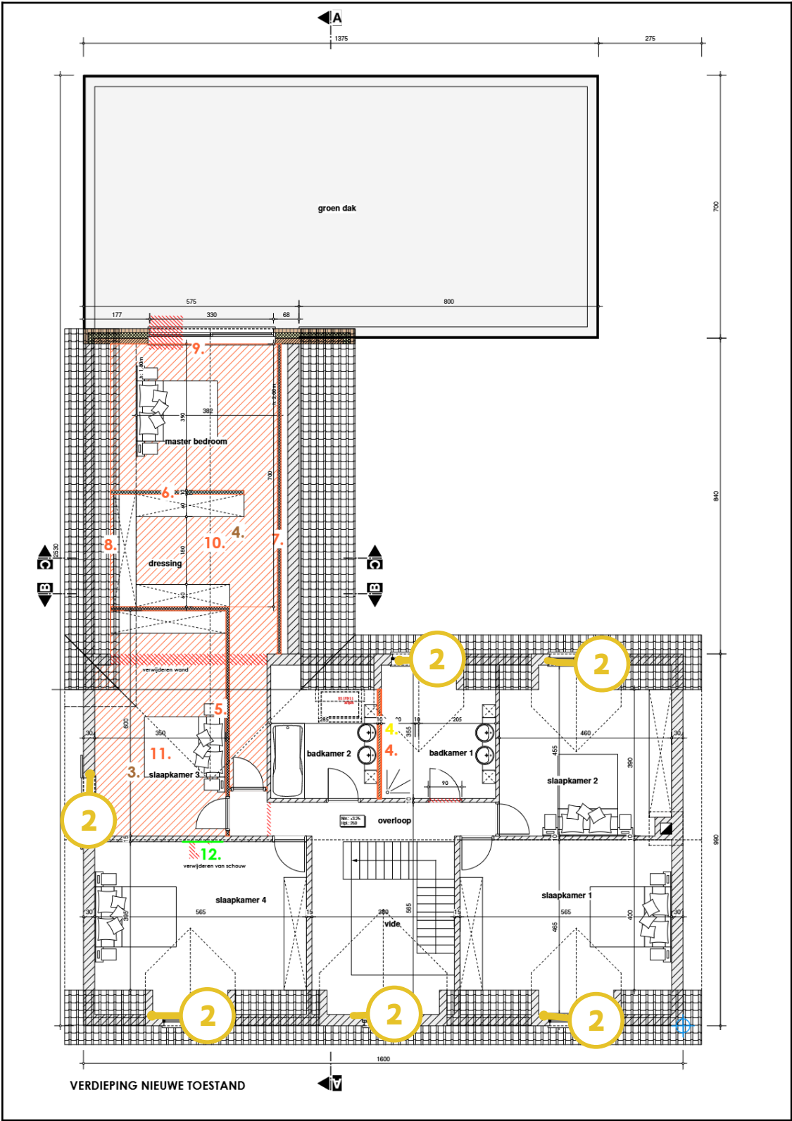
Legende van plan 1.9: afwerking - verdieping
