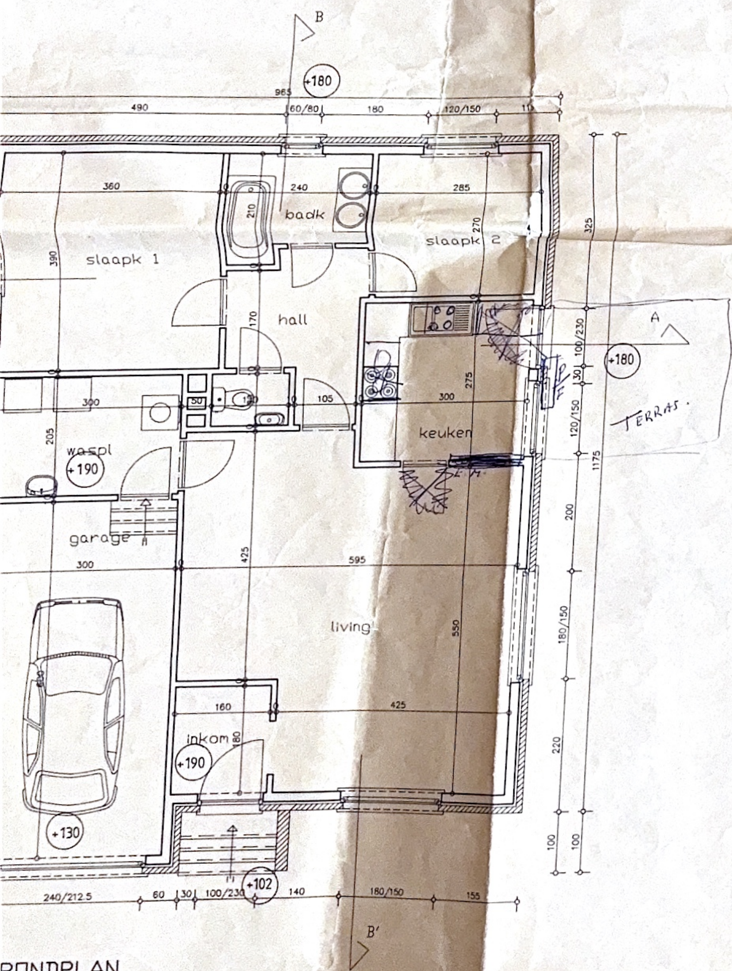
GRONDPLAN
