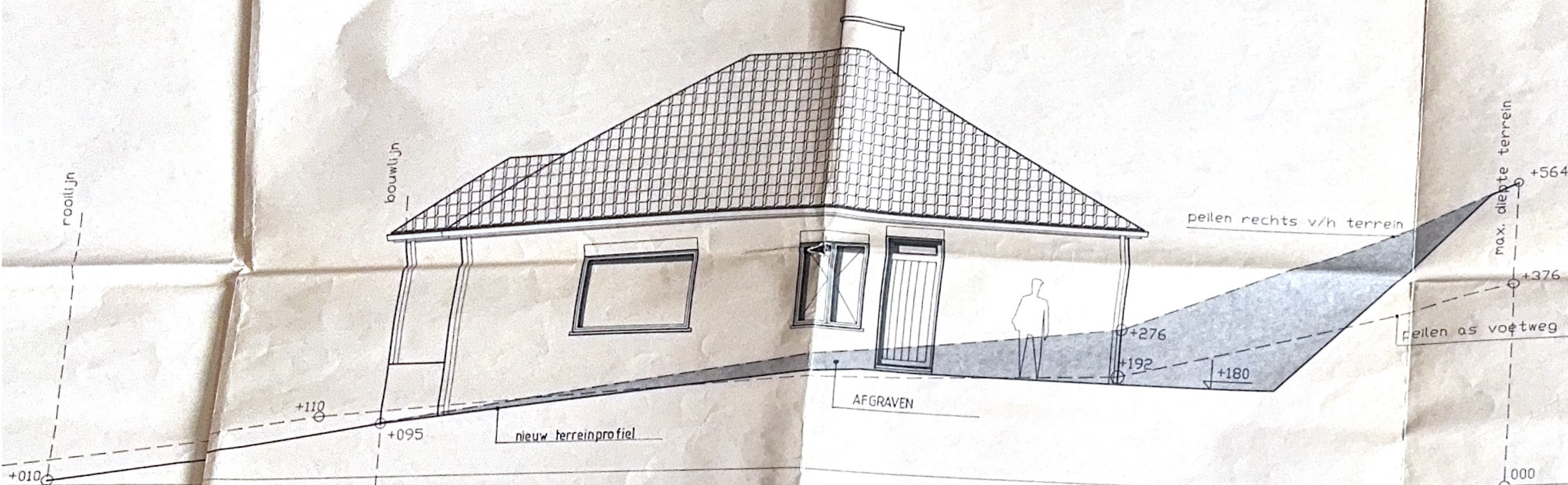
ZIJGEVEL RIJTS
