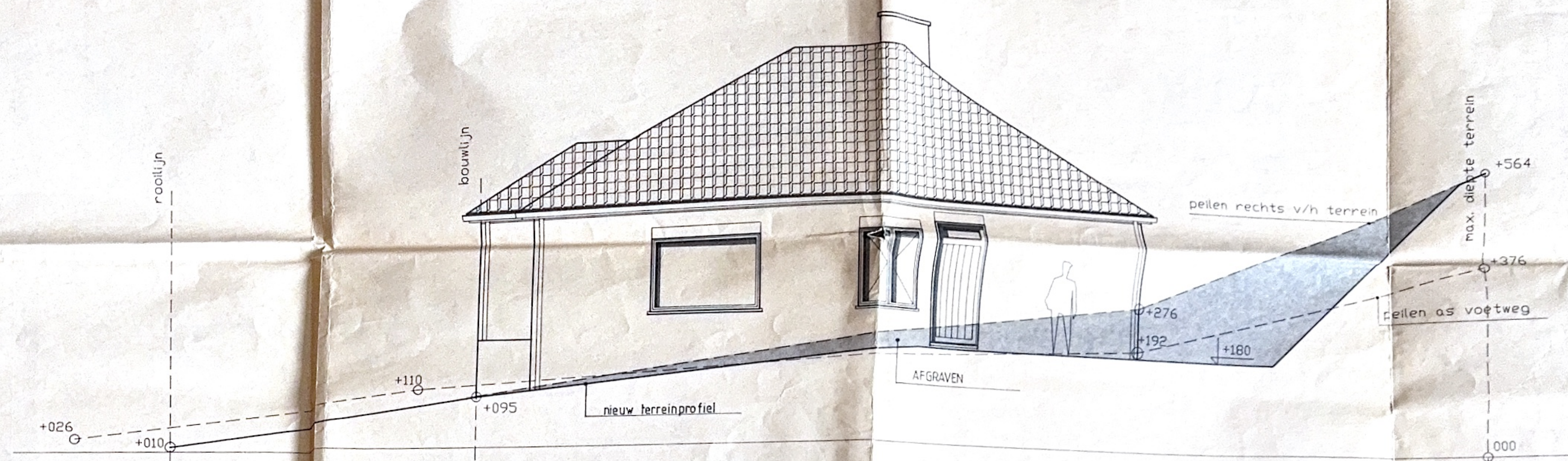
ZIJGEVEL RECHTS
