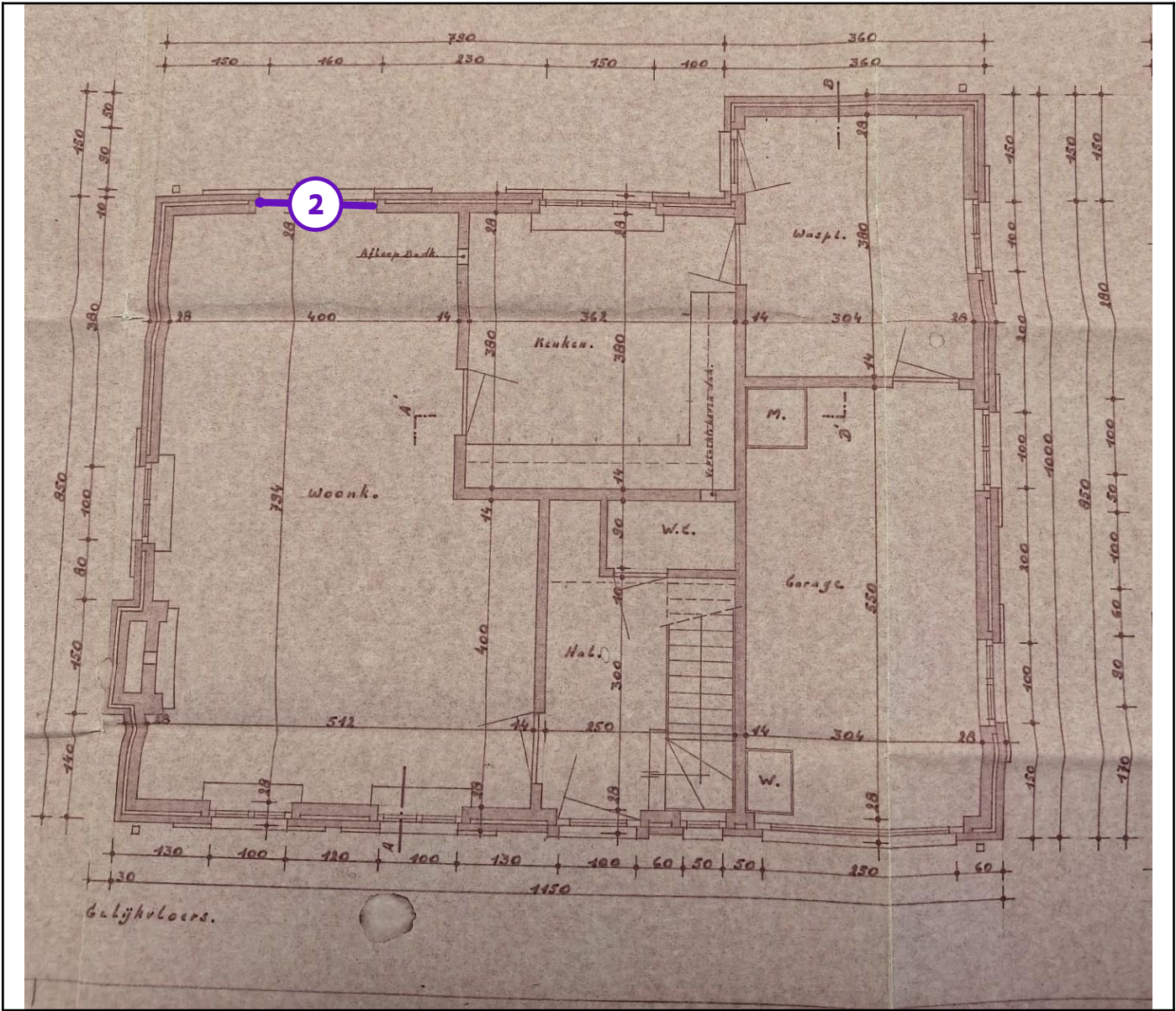
Legende van plan 1.6: Plan Gelijkvloers
