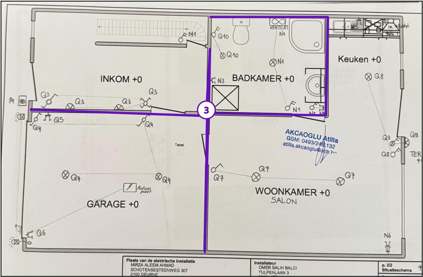
Legende van plan 1.8: Gelijkvloers
