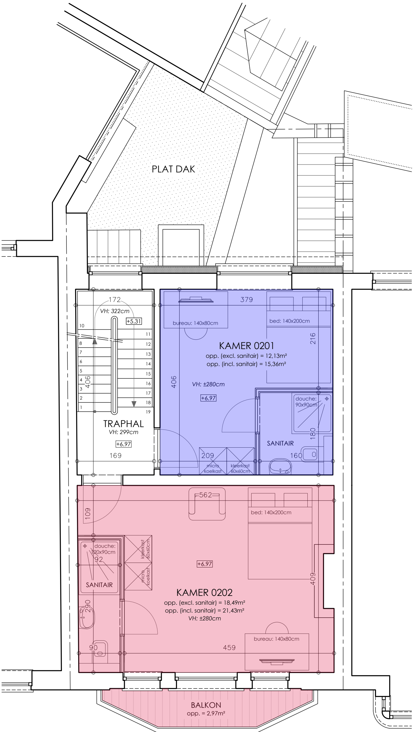
VERDIEPING 2
