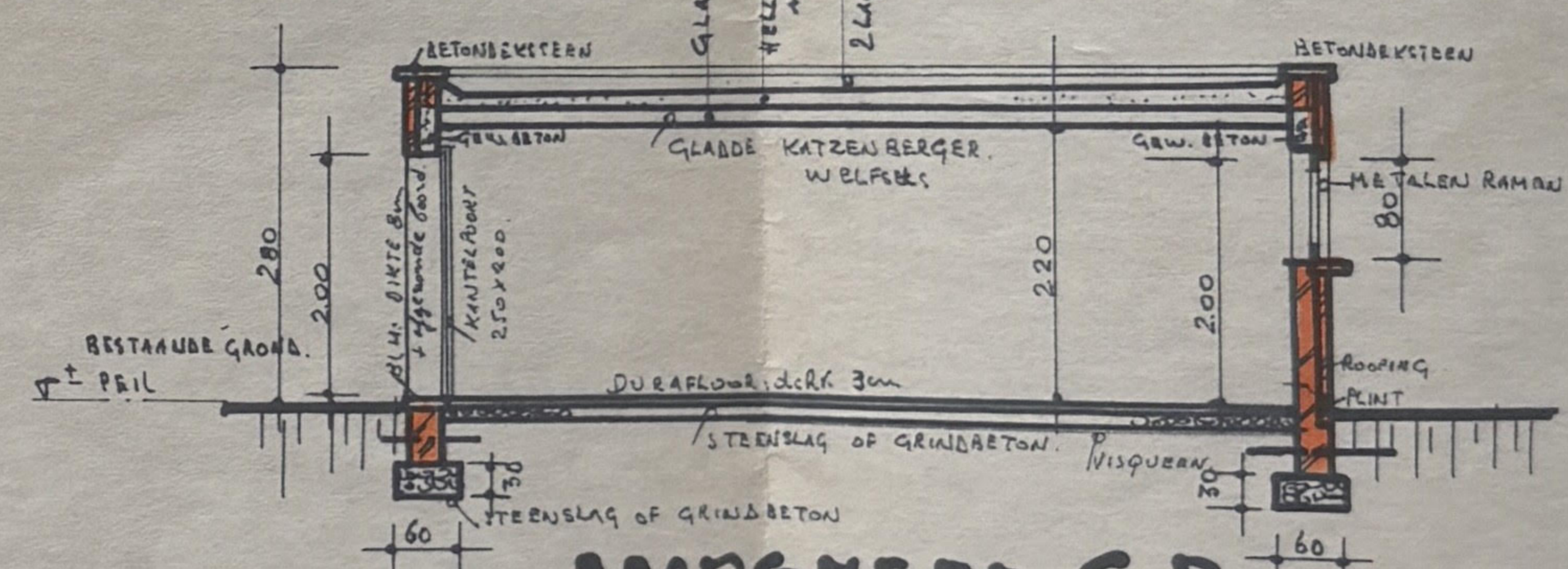
DOORSNEDEN C-D.
