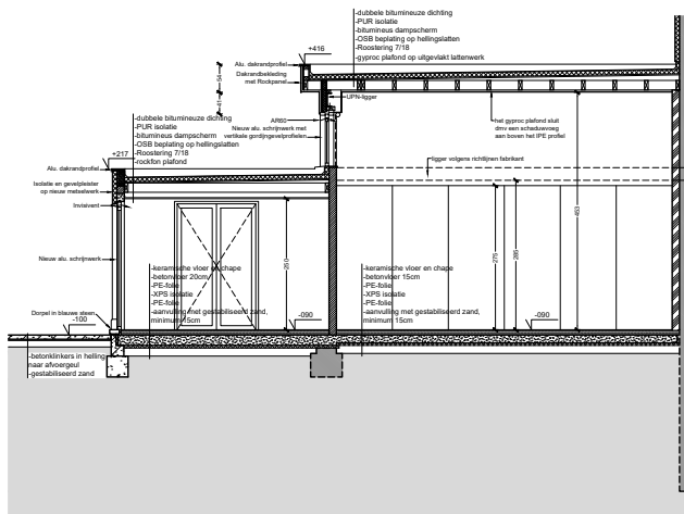
Doorsnede DD Nieuwe Situatie
