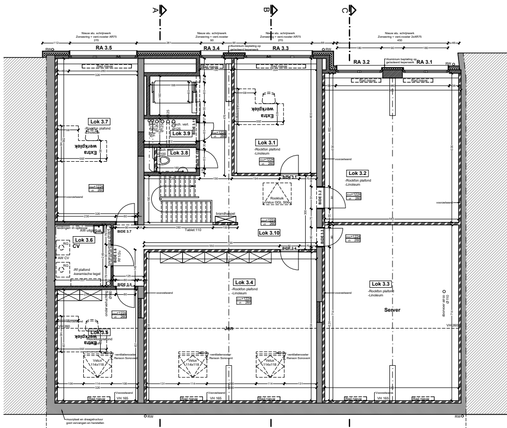
Verdieping 3 Nieuwe Situatie
