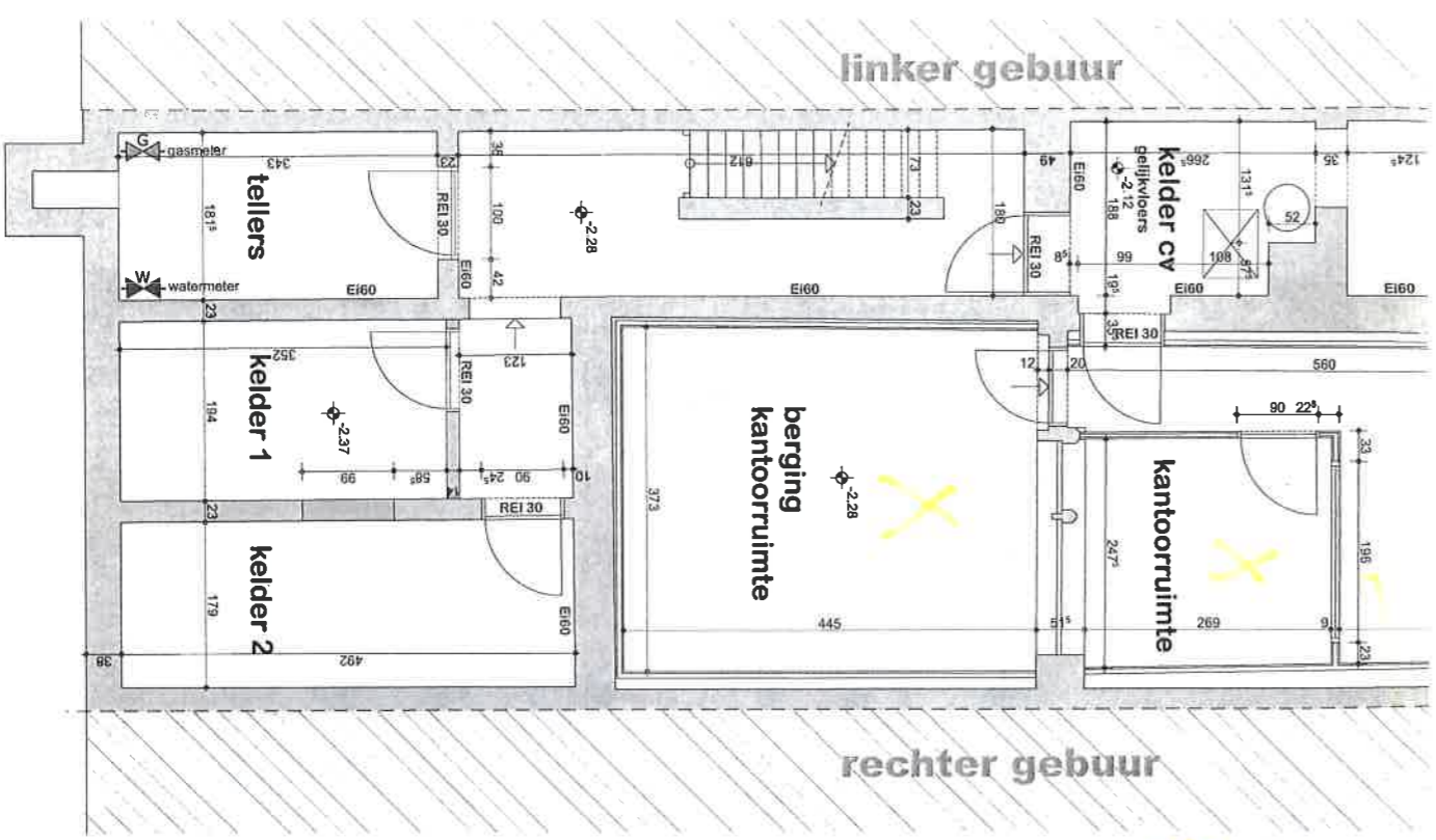
Kelderplan schaal 1-50
