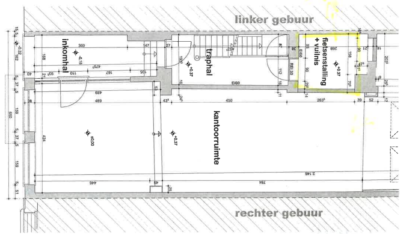
gelijkvloers schaal 1-50
