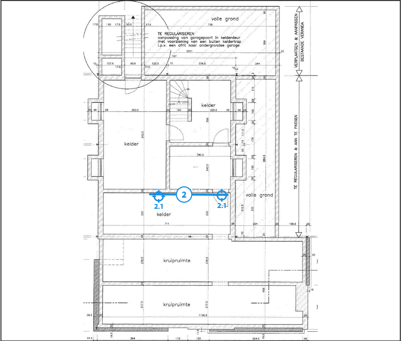
Legende van plan 1.1: Kelderplan
