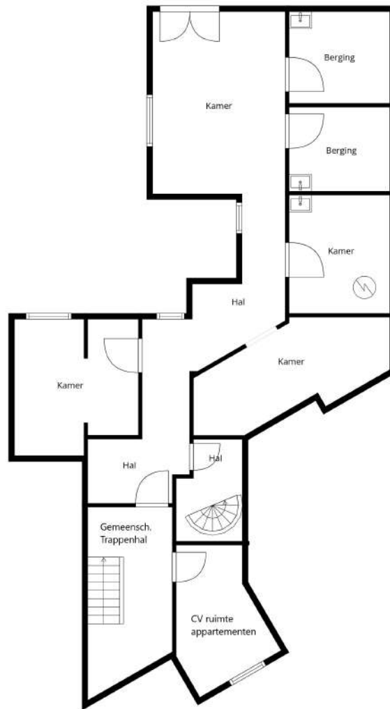
KELDERVERDIEPING
