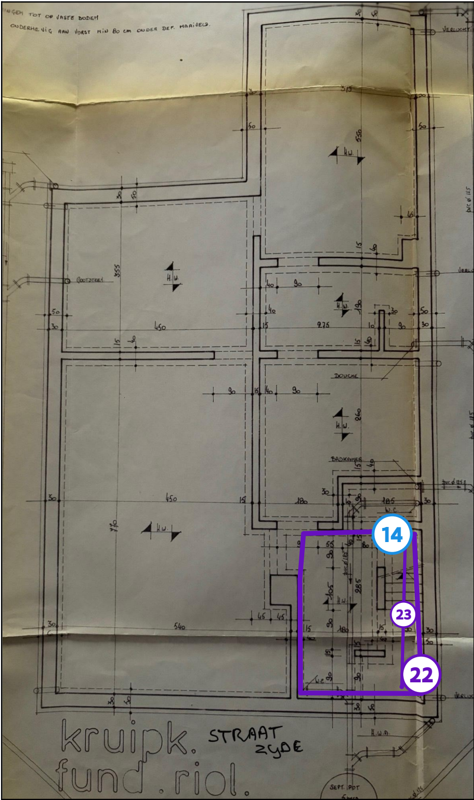
Legende van plan 1.2: Kelder
